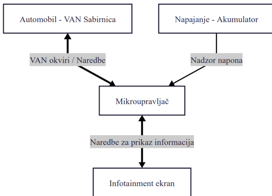
Slika 2.10. Osnovni blok dijagram programskog rješenja.
