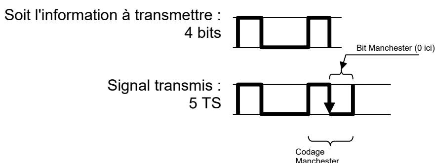
Slika 2.1. e-Manchester kodiranje. [1]
