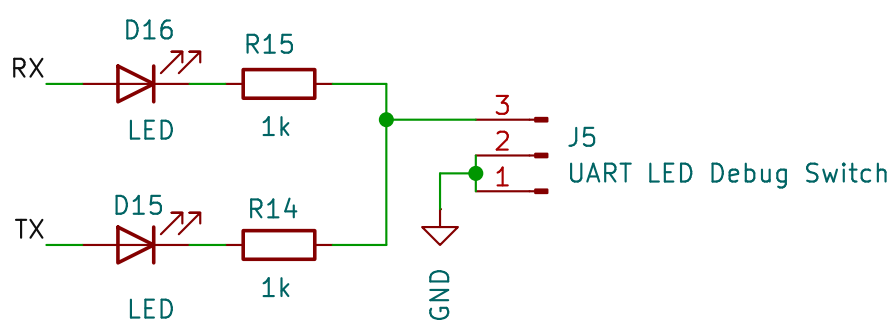
Slika 3.16. Pregled sheme - LE diode za detekciju i otklanjanje grešaka na UART sabirnici.
