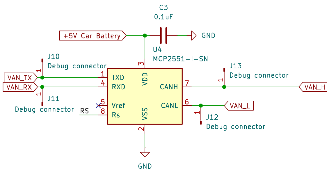
Slika 3.10. Pregled sheme - MCP.
