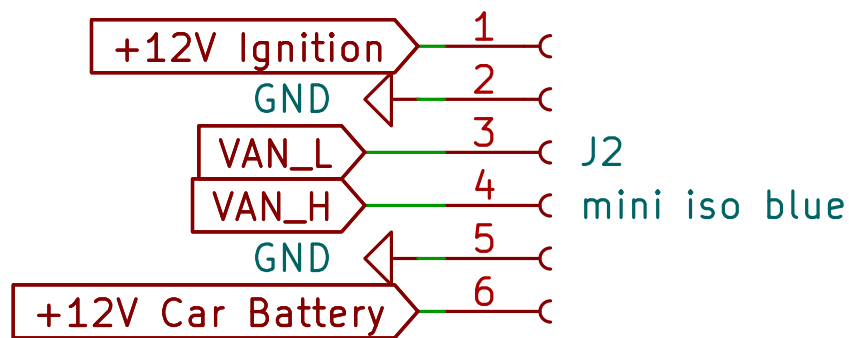
Slika 3.22. Pregled sheme - Spojnica za VAN mrežu automobila.
