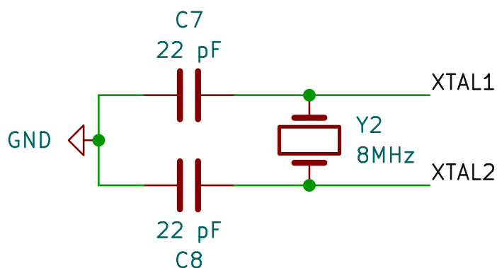
Slika 3.7. Pregled sheme - TSS oscilator.
