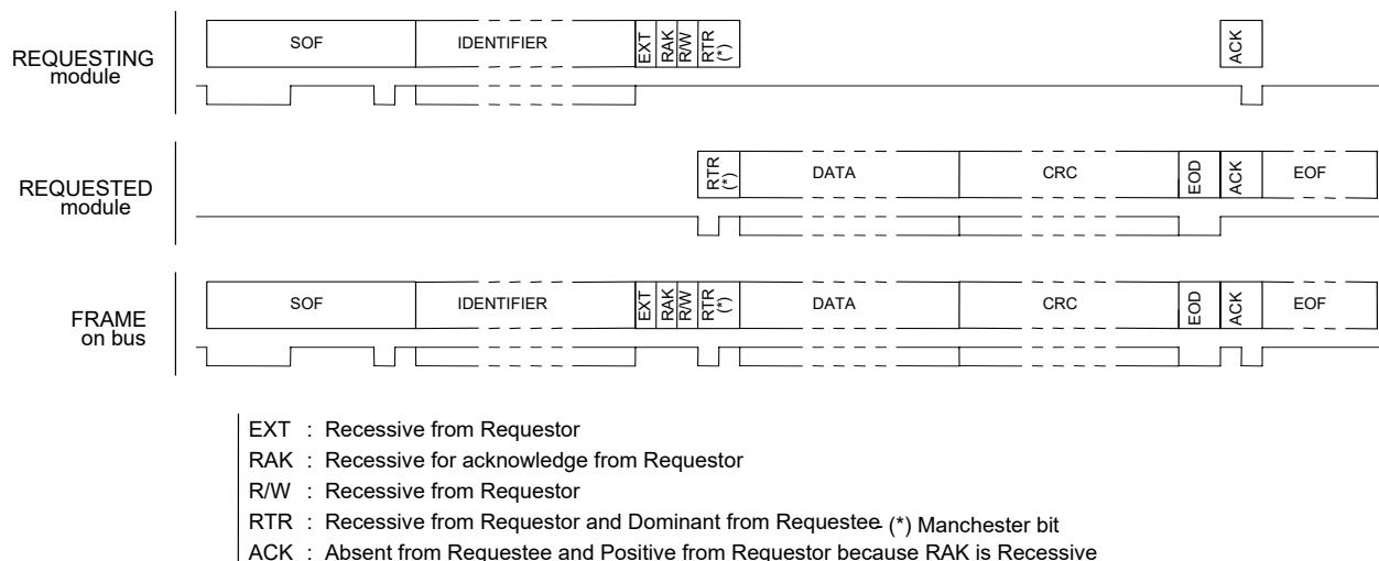
Slika 2.6. Ilustracija prijena zahtjeva s trenutnim odgovorom. [3]
