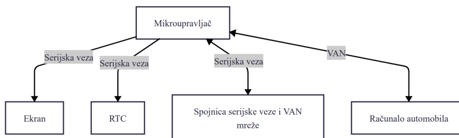
Slika 2.9. Osnovni blok dijagram sklopovskog rješenja.
