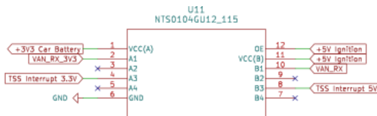
Slika 3.5. Pregled sheme - pretvarač naponskih razina A
