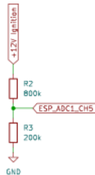
Slika 3.14. Pregled sheme - Djeliteľ napona baterije
