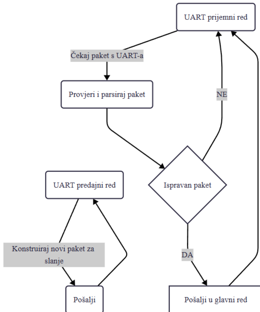
Slika 3.28. Blok dijagram programskog toka – UART red
