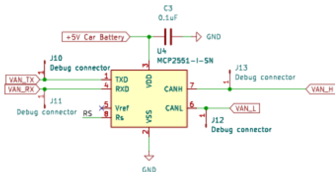
Slika 3.10. Pregled sheme - MCP
