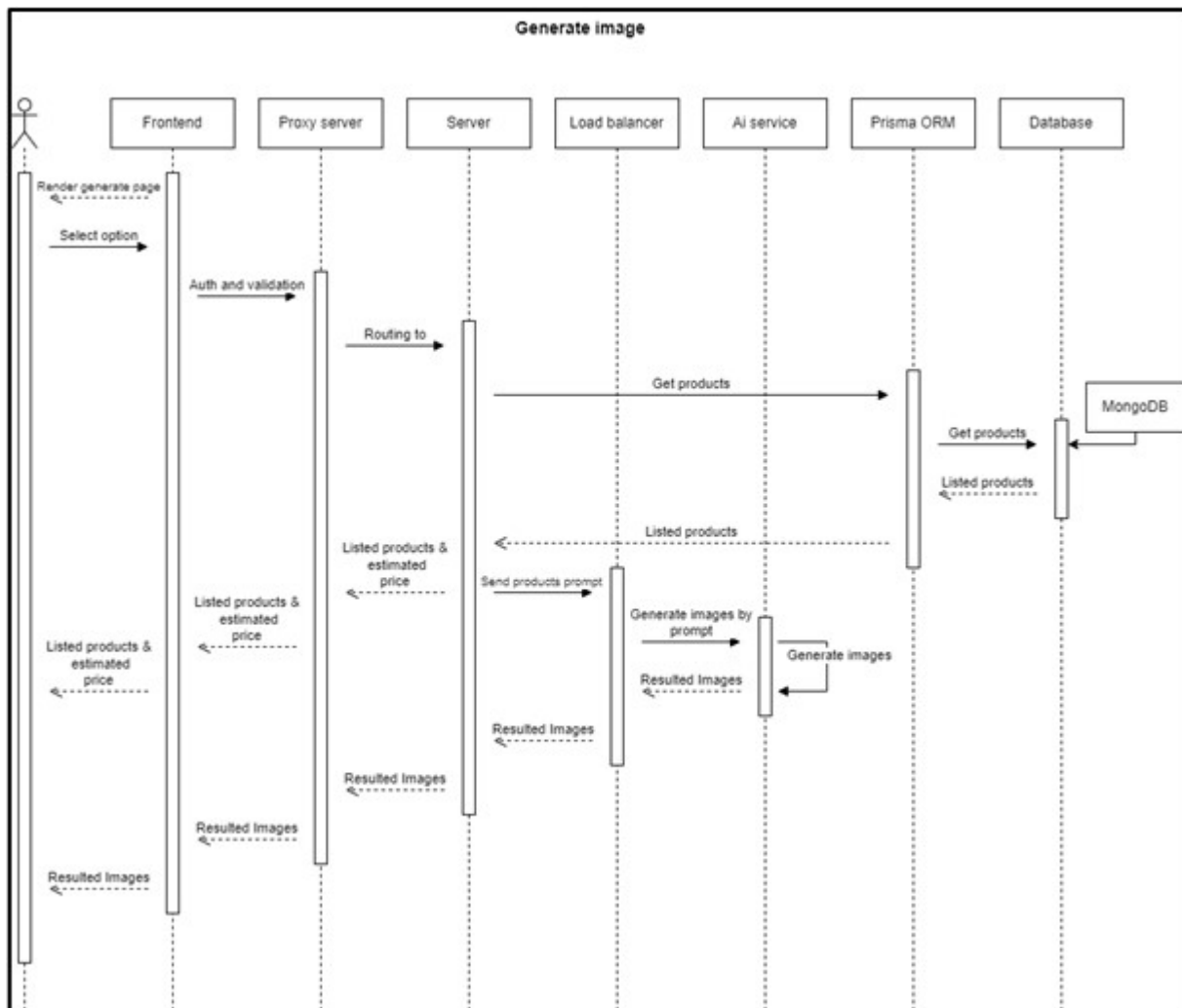
รูปที่ 3.10 Sequence Diagram
