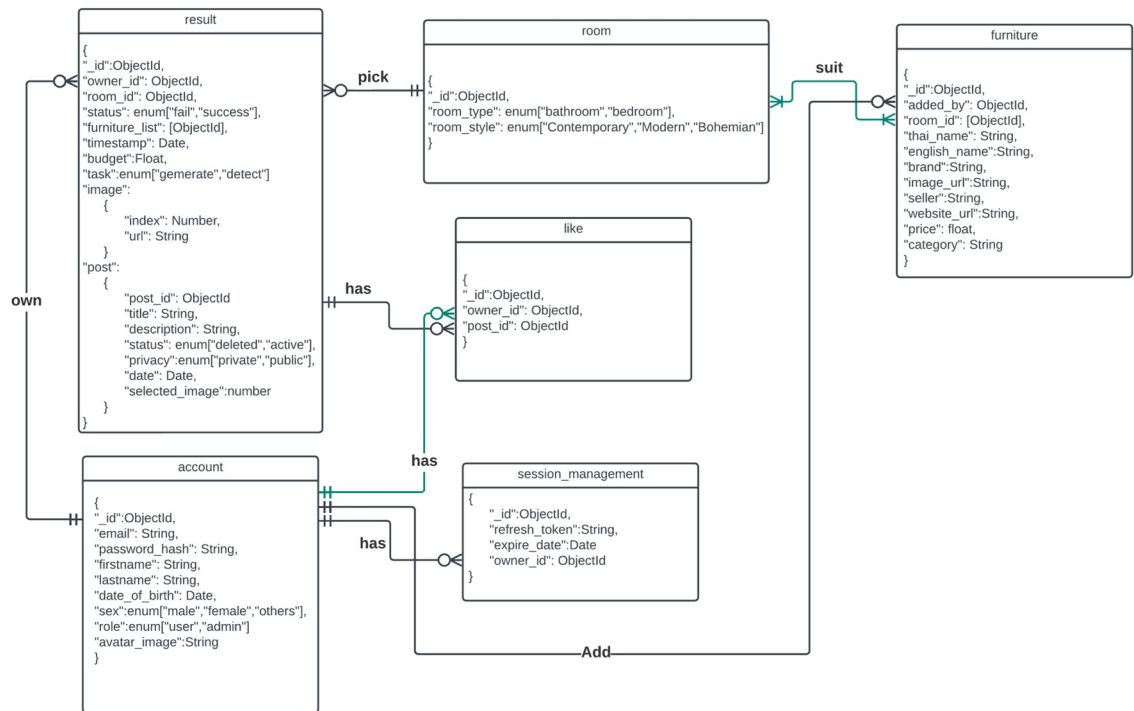
รูปที่ 3.12 ER Diagram
