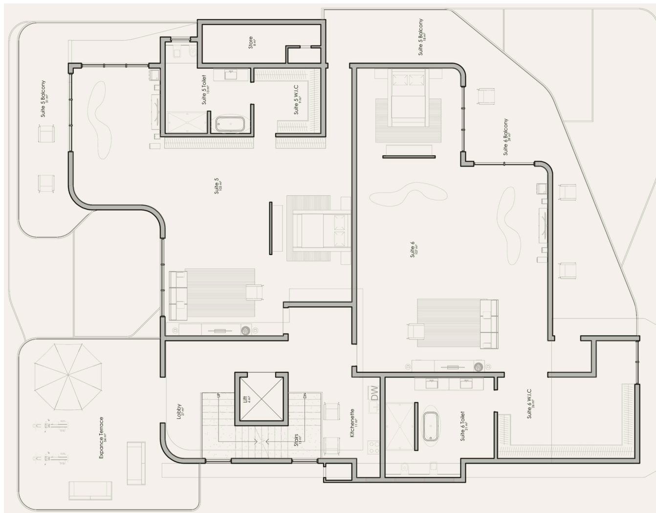
SECOND FLOOR · N.T.S
