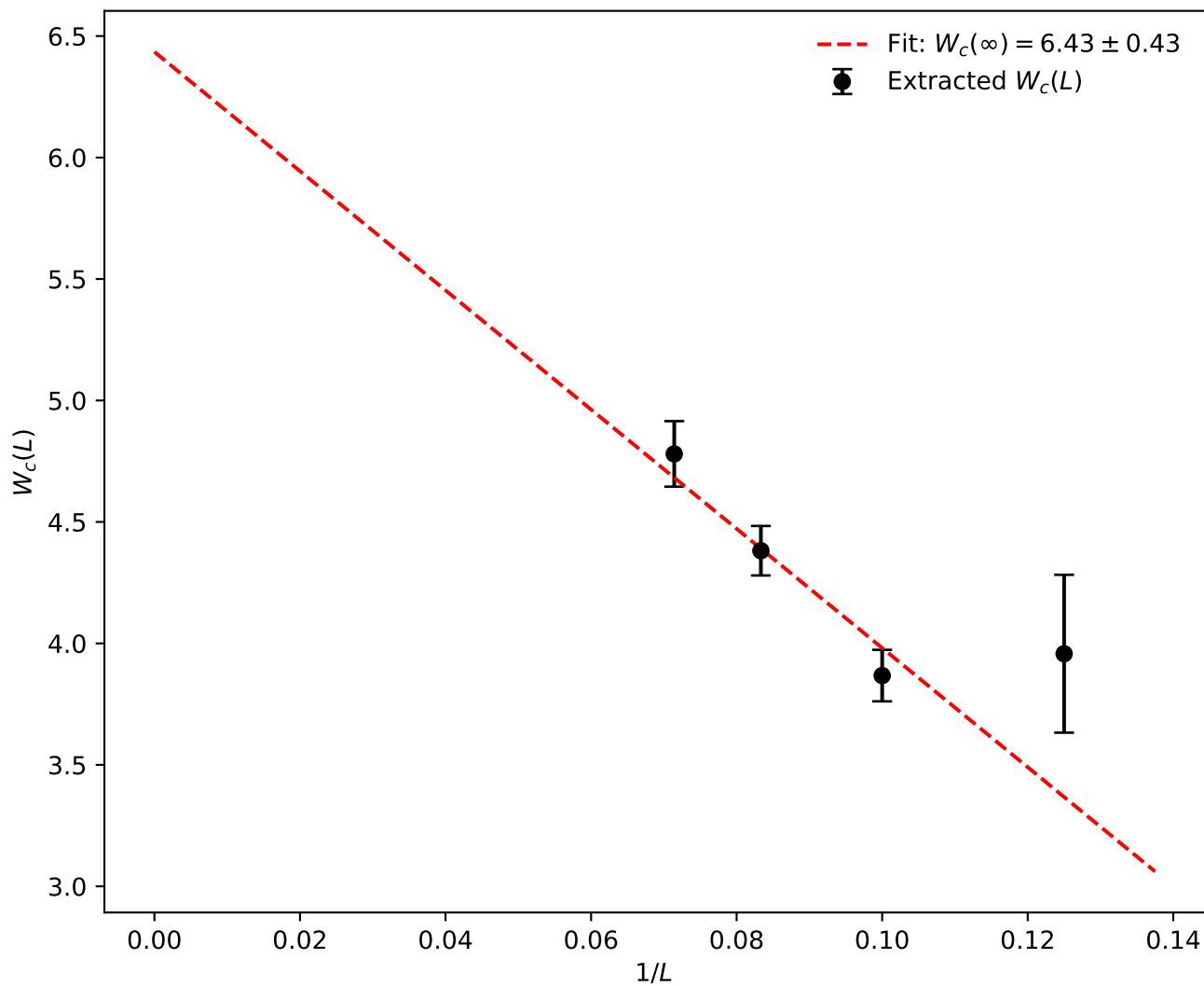
Finite-Size Scaling ( J_2 = 0.5 )
