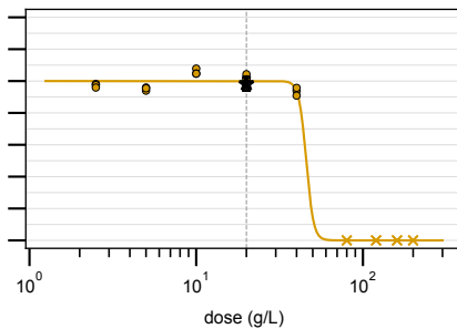
lactic acid (LA)
