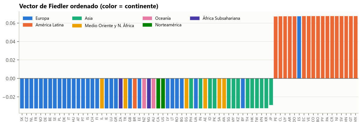
Figura 3: Vector de Fiedler ordenado, coloreado por continente.
