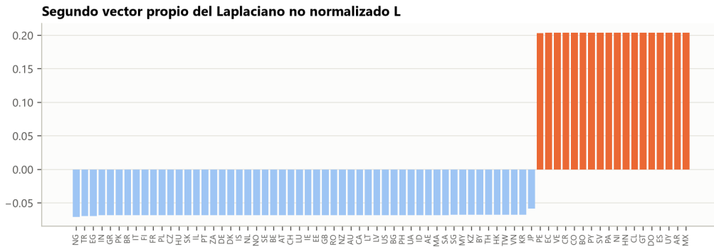
Figura 7: Segundo vector propio del Laplaciano no normalizado.
