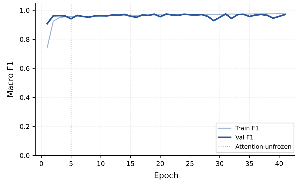
CNN+Attention — Macro F1
