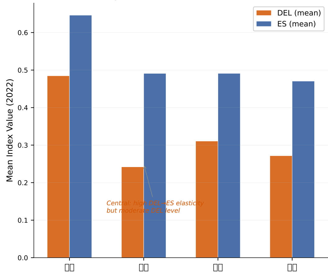
Regional Mean DEL & ES (2022)
