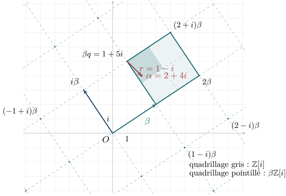
Figure 16.2: Le quadrillage carré usuel \mathbb{Z}[i] et, superposé, le quadrillage \beta\mathbb{Z}[i] pour \beta = 3 + 2i . Le point \alpha = 2 + 4i appartient à une cellule du nouveau réseau ; son sommet le plus proche est le multiple \beta q = 1 + 5i . Le petit vecteur r = \alpha - \beta q = 1 - i est le reste de la division euclidienne.
