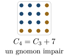
Figure 1.3: Deux façons de voir une formule : T_n - T_{n-1} = n et C_n - C_{n-1} = 2n - 1 . Les points ocre sont ceux que l'on ajoute.
