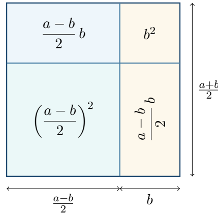
Figure 13.2: Décomposition du carré de côté (a+b)/2 .
