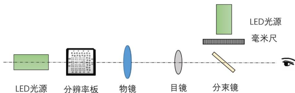
图 4.3 测显微镜视角放大率实际光路图（人眼紧贴分束镜观察）
