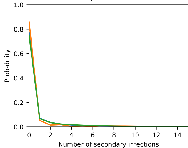
Negative Binomial
