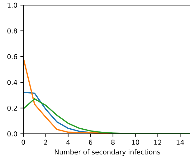
Poisson
