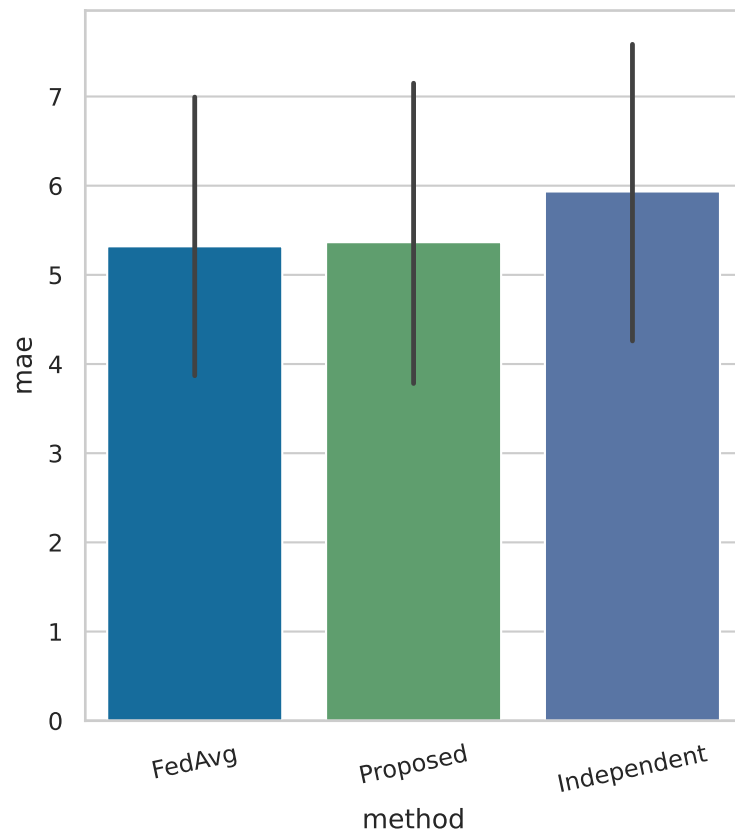
MAE
