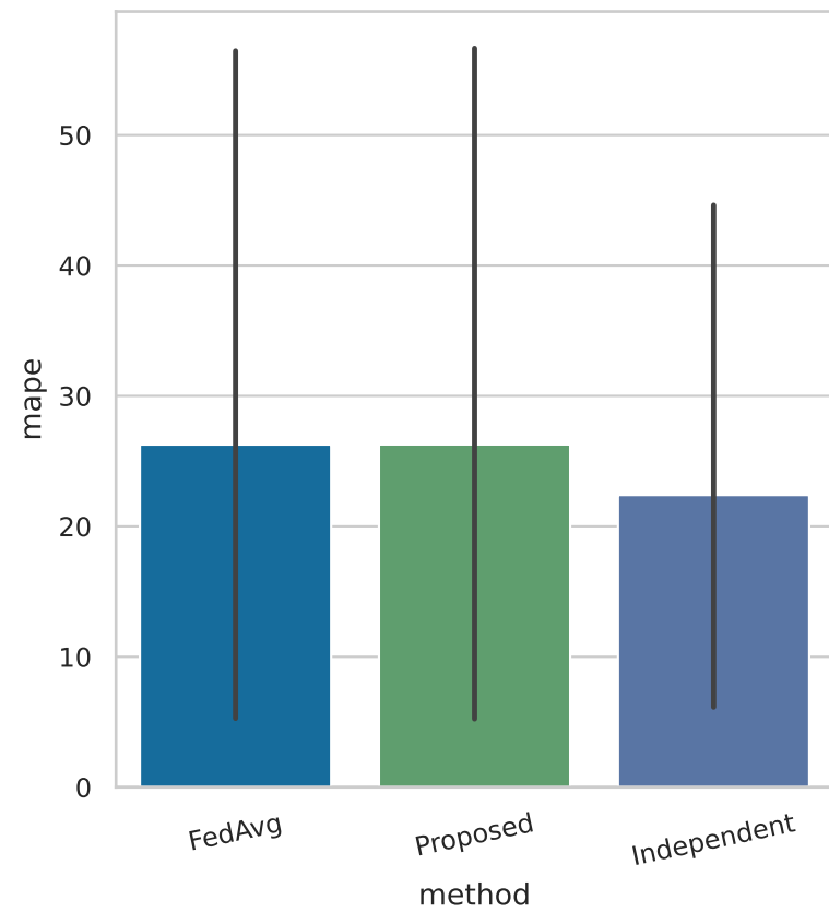
MAPE
