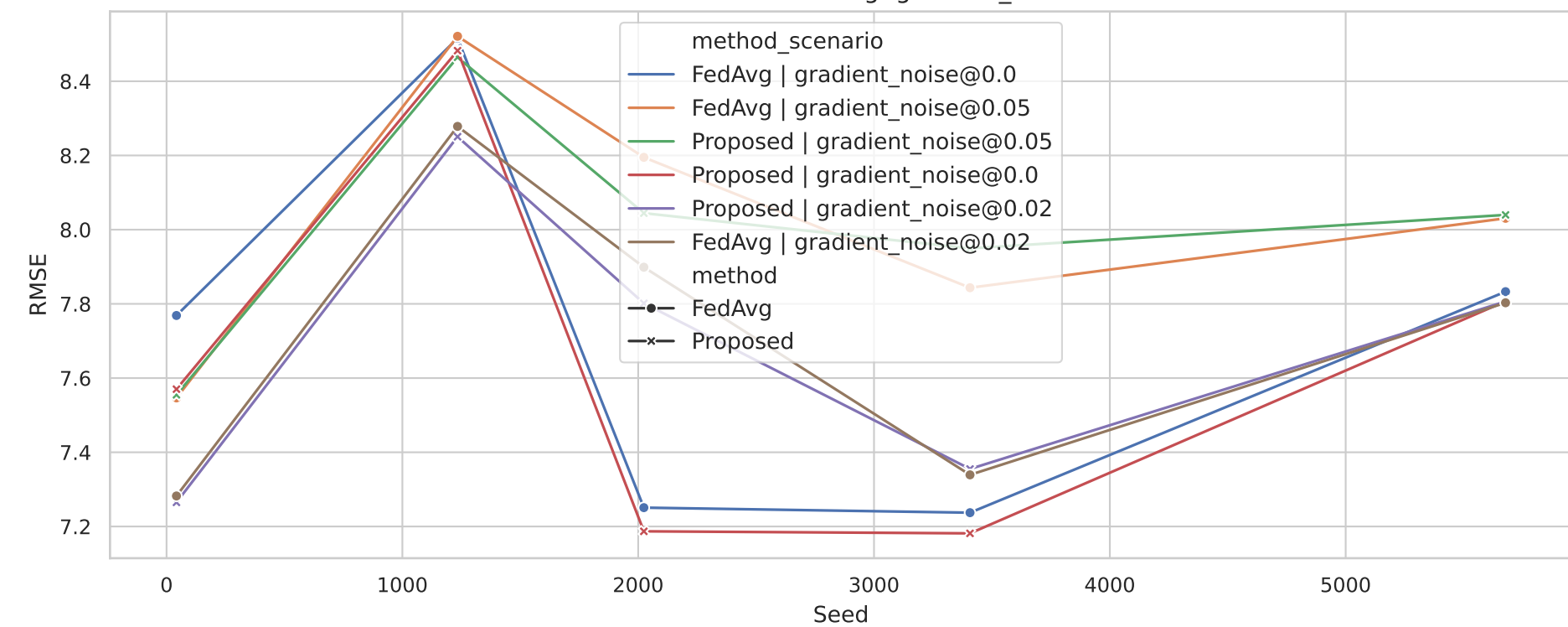
Per-seed RMSE Pairing: gradient_noise
