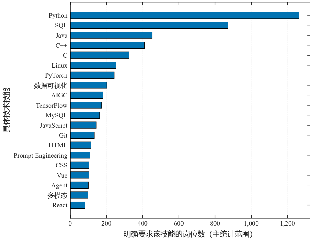
图05 核心技术技能 Top20 (主统计范围 REQUIREMENT_SECTION, 分母 8,822 个岗位)
