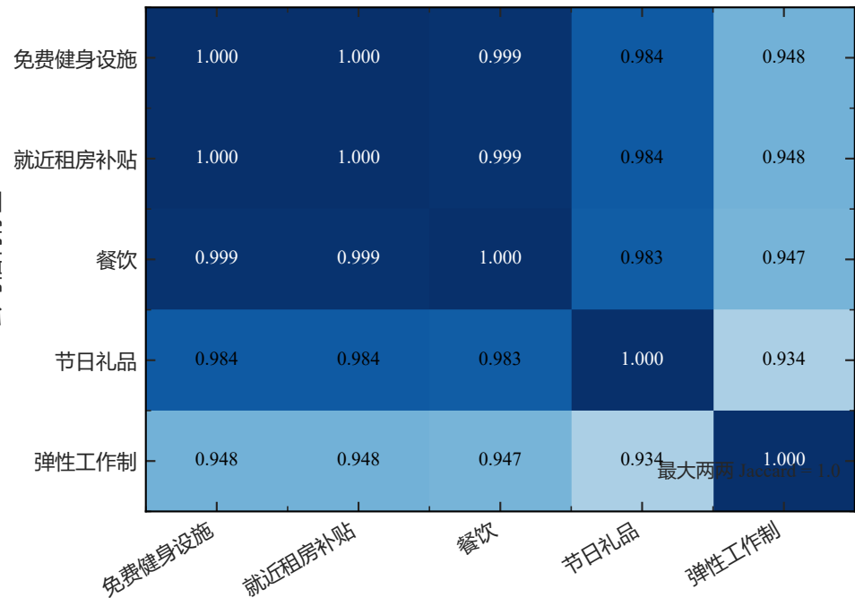
(b) 前 5 标签两两 Jaccard 热力图
