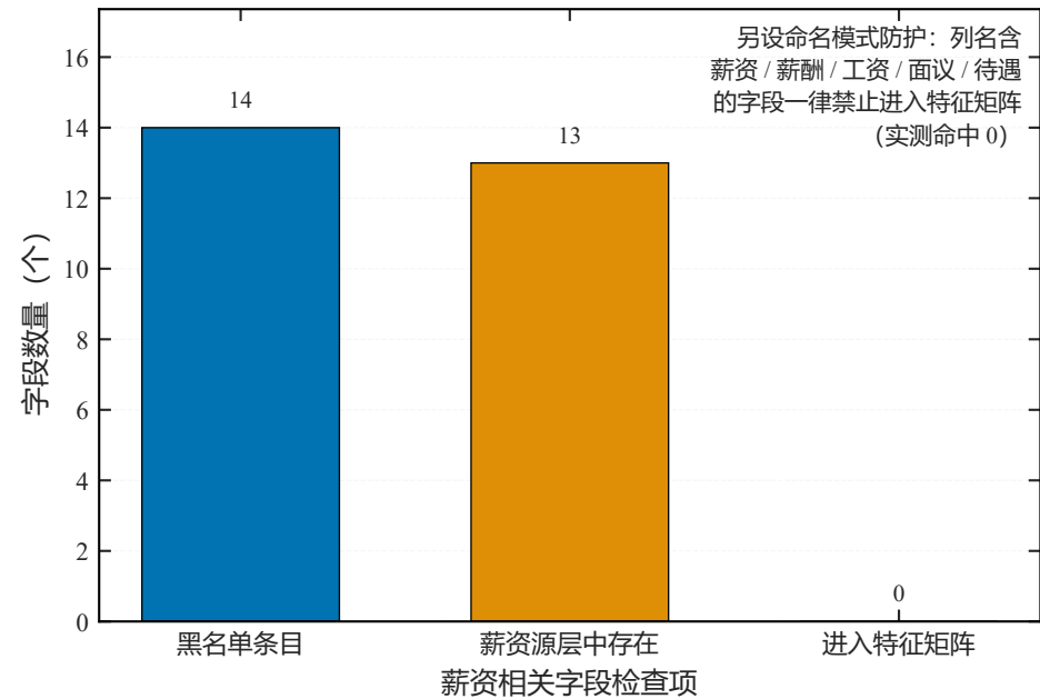
(a) 泄漏字段检查状态
