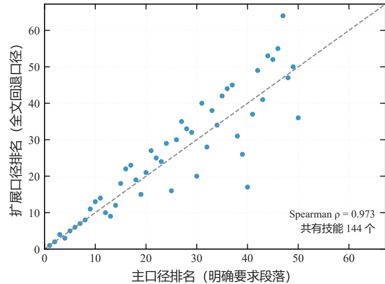
(a) 双口径技能排名对照 (Top50)
