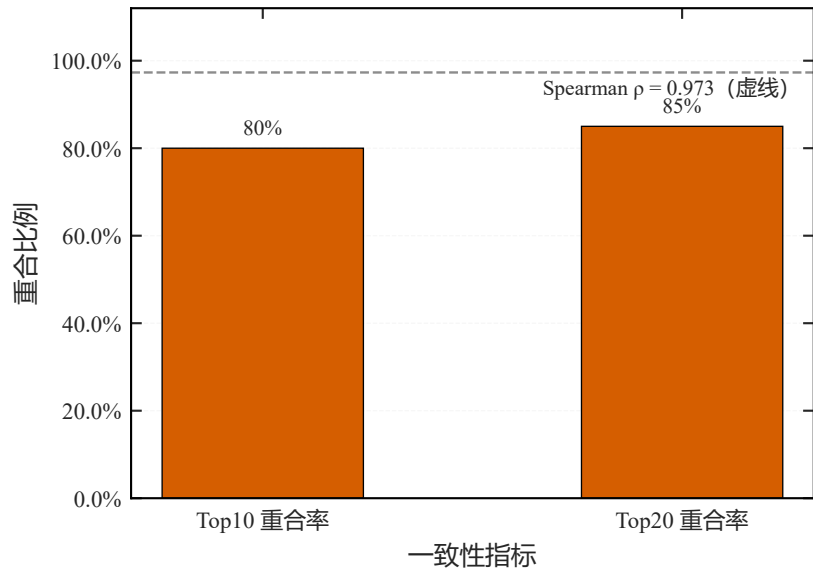
(b) Top-K 重合率与排名相关
