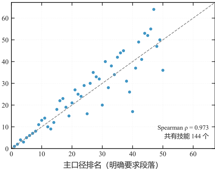
(a) 双口径技能排名对照 (Top50)
