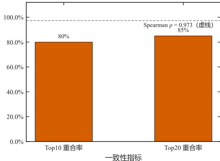
(b) Top-K 重合率与排名相关
