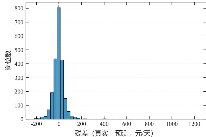
(a) 残差分布 (虚线为中位数)
