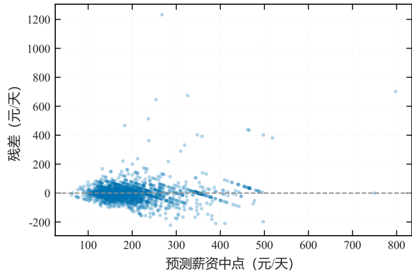
(b) 残差 vs 预测值
