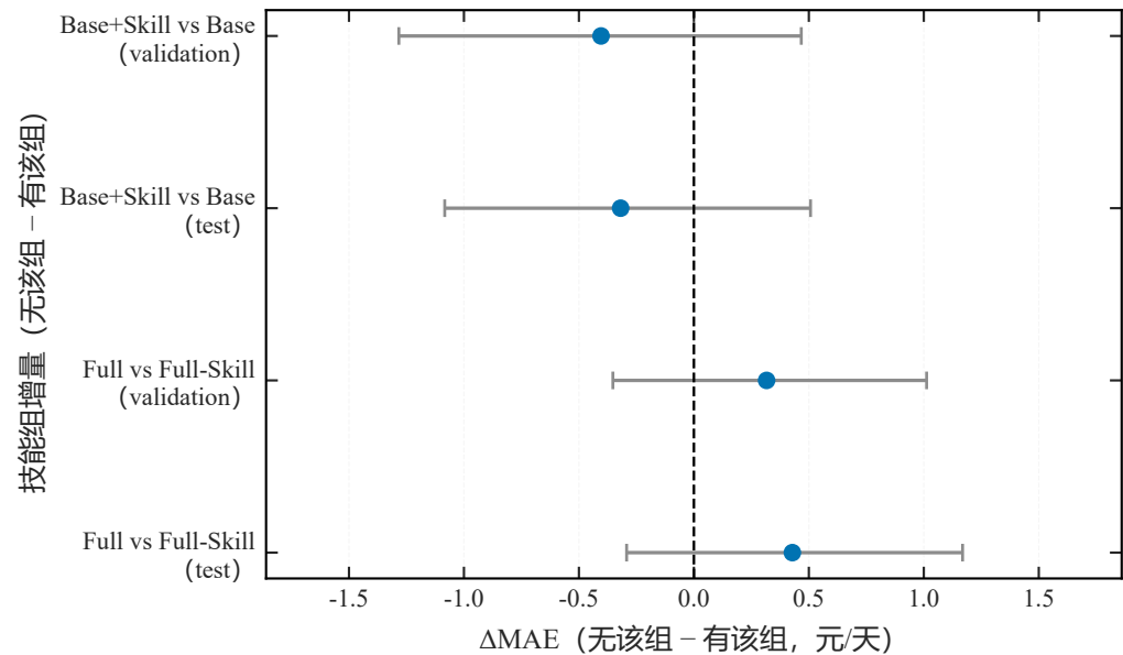
(b) 技能增量 \Delta MAE 与 bootstrap 95% 置信区间
