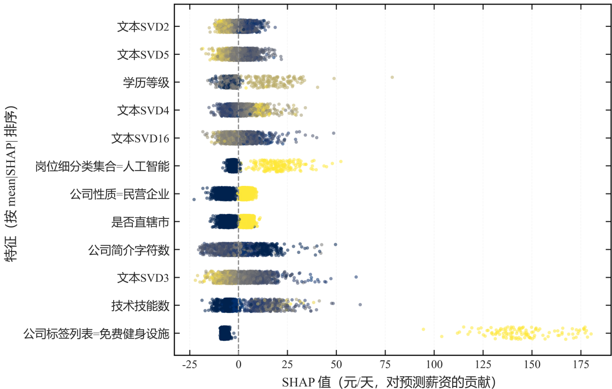
图 8-3 正式主模型 SHAP 蜂群图 (Top12 特征)
