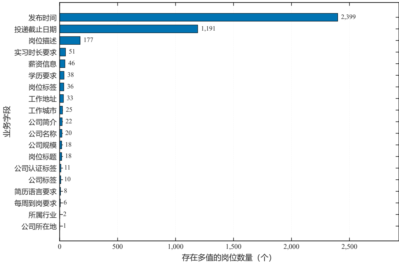
图09 业务字段组内冲突岗位数量
