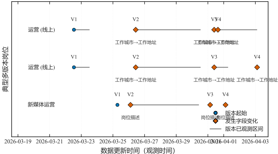
图15 典型岗位核心业务版本演化时间轴
