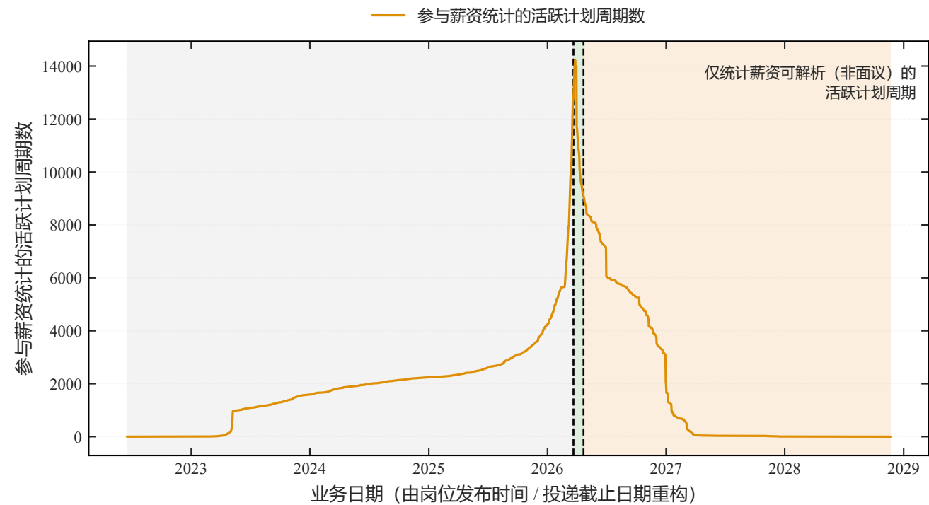
(b) 每日参与薪资统计的活跃计划周期数 (读图可靠性)
