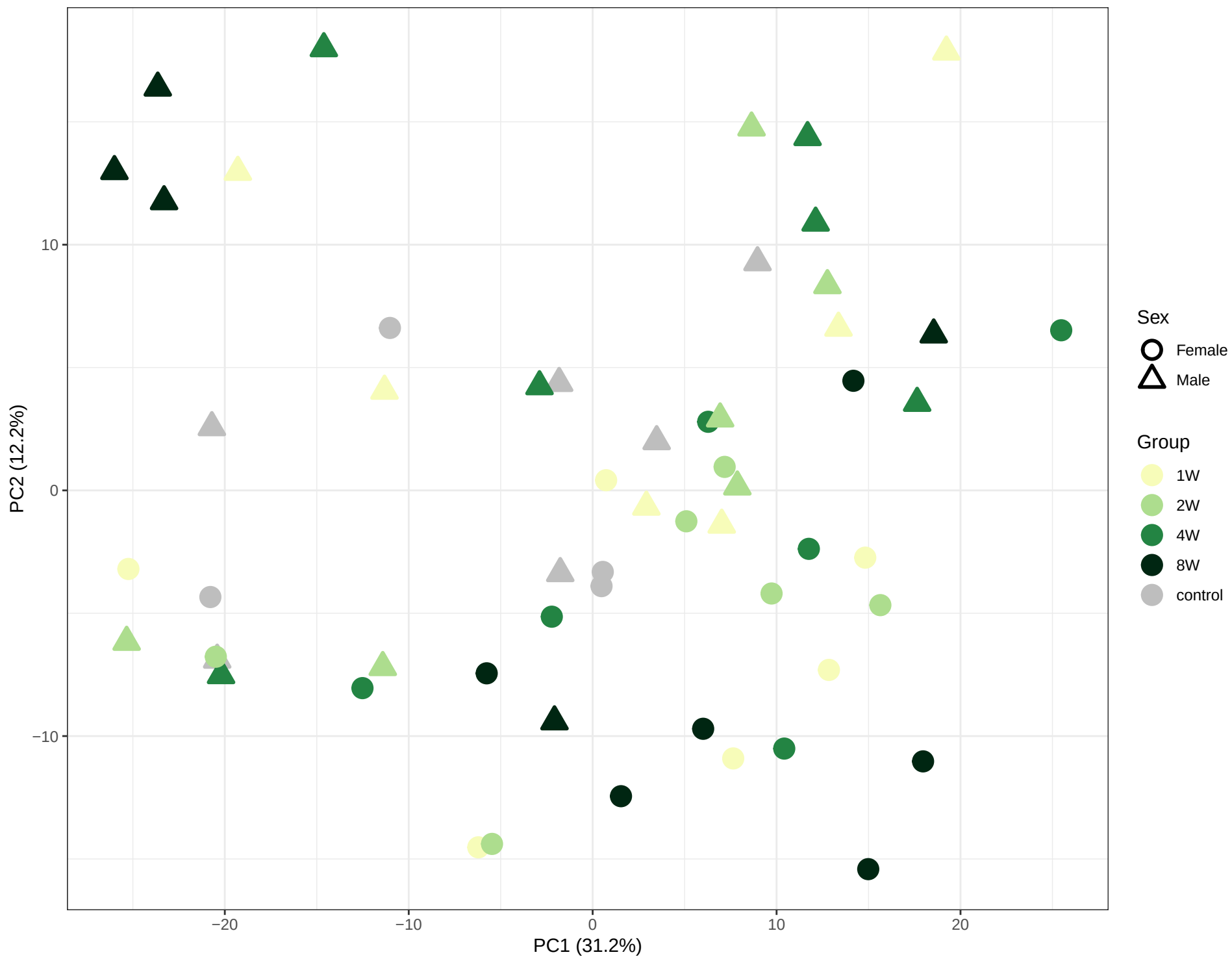
REDOX_GN_NORM PCA
