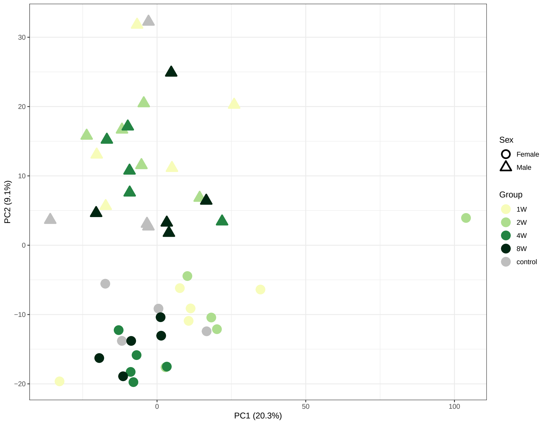
TRNSCRIPT_VL PCA
