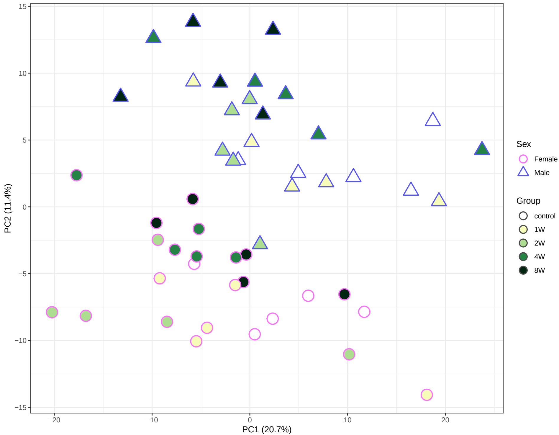
METAB_GN PCA
