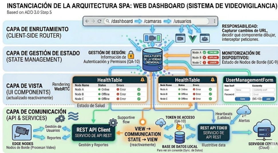
Figura 5: Patrón SPA Instanciado
