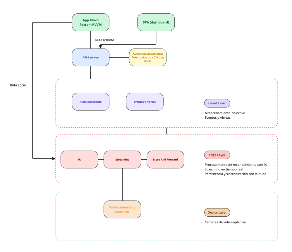
Figura 4: Arquitectura Edge Computing instanciada
