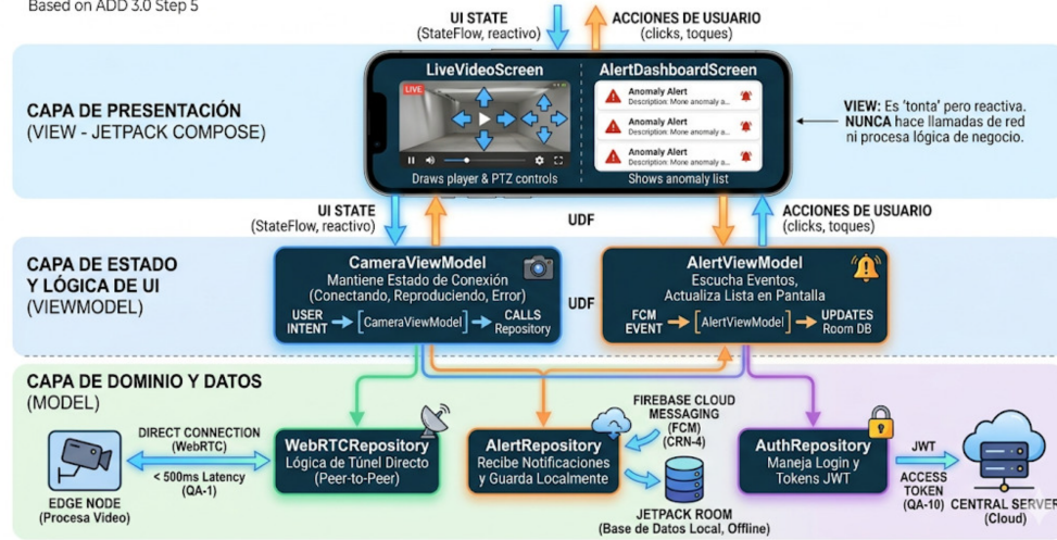
Figura 6: Patrón MVVM Instanciado
