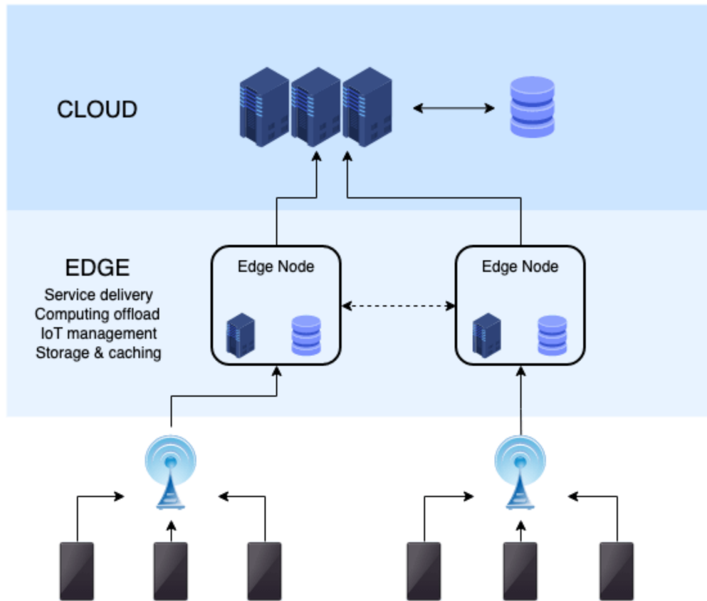
Figura 1: Arquitectura Edge Computing
