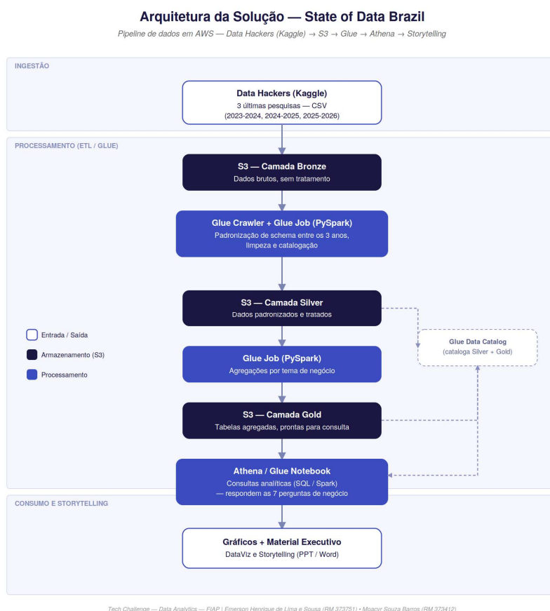
Figura 1 — Diagrama de arquitetura da solução (mesmo conteúdo do arquivo .drawio anexo).
