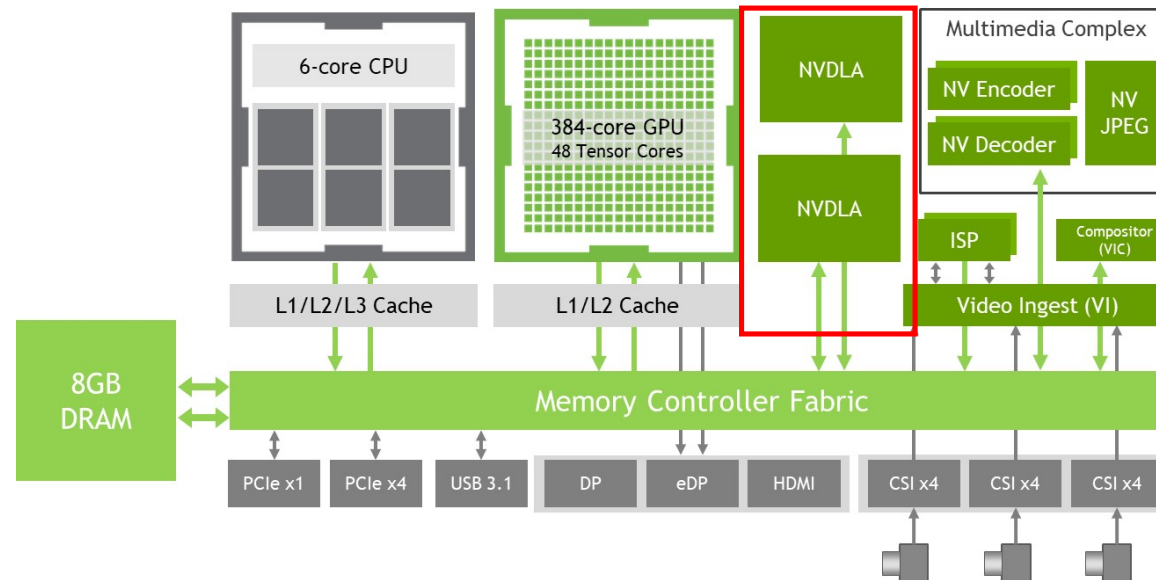
NVIDIA Jetson Xavier
