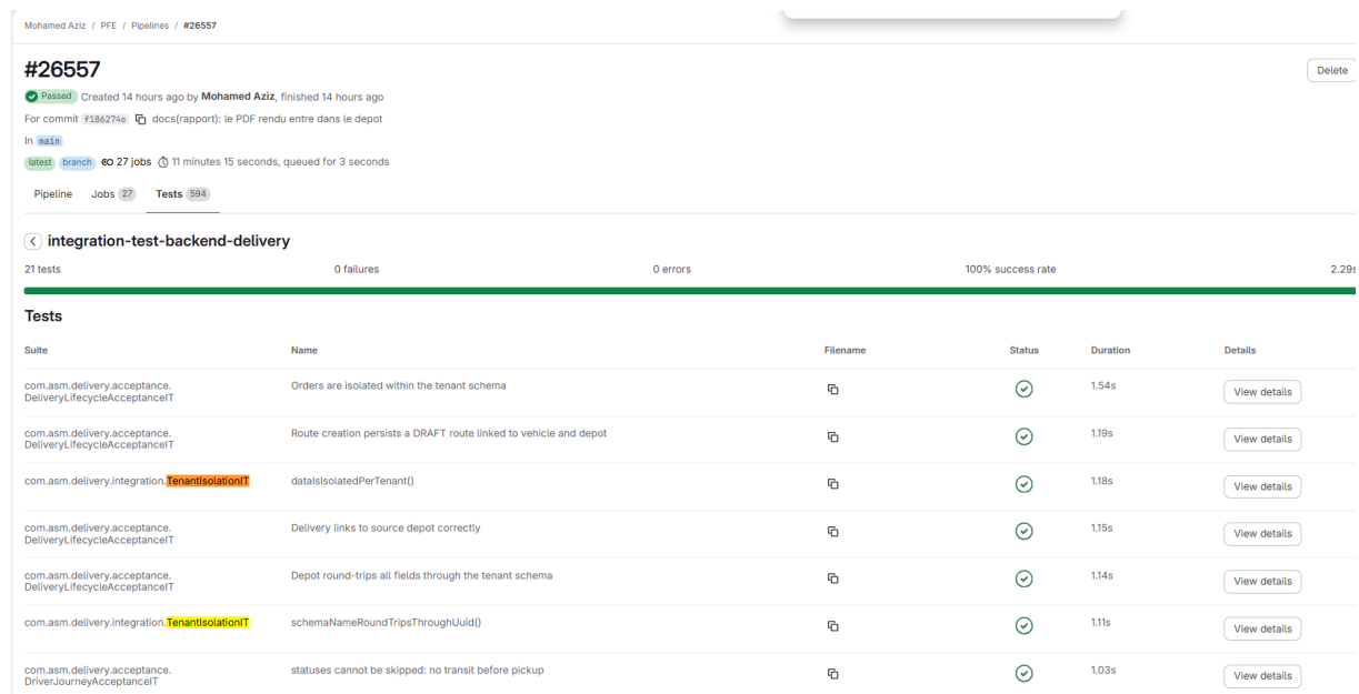
FIG. 4.12 : Exécution en CI des tests d'isolation
