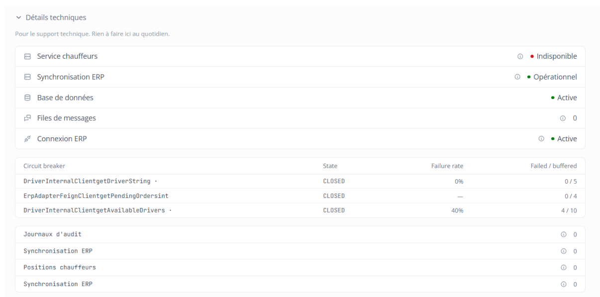
FIG. 8.7 : Volet «Détails techniques» : composants, disjoncteurs et files de rebut
