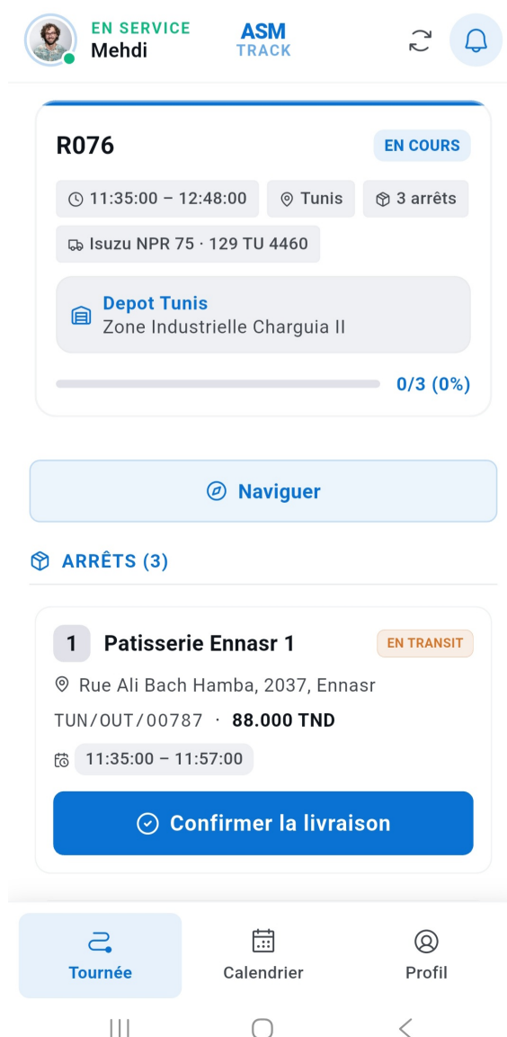
FIG. 7.4 : Tournée du jour sur l'application chauffeur
