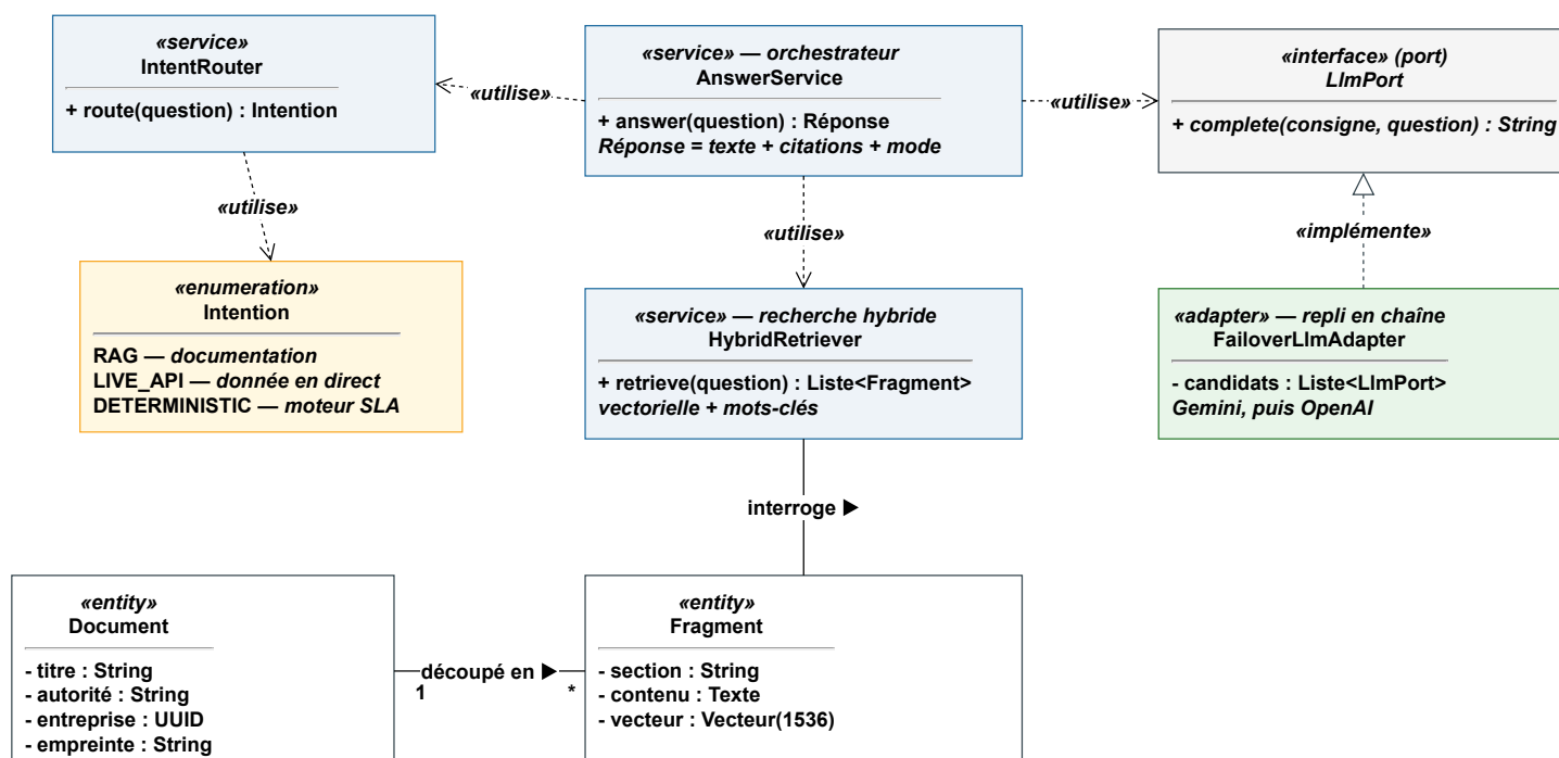
FIG. 8.4 : Classes de l'assistant : routage, recherche hybride et port vers le modèle
