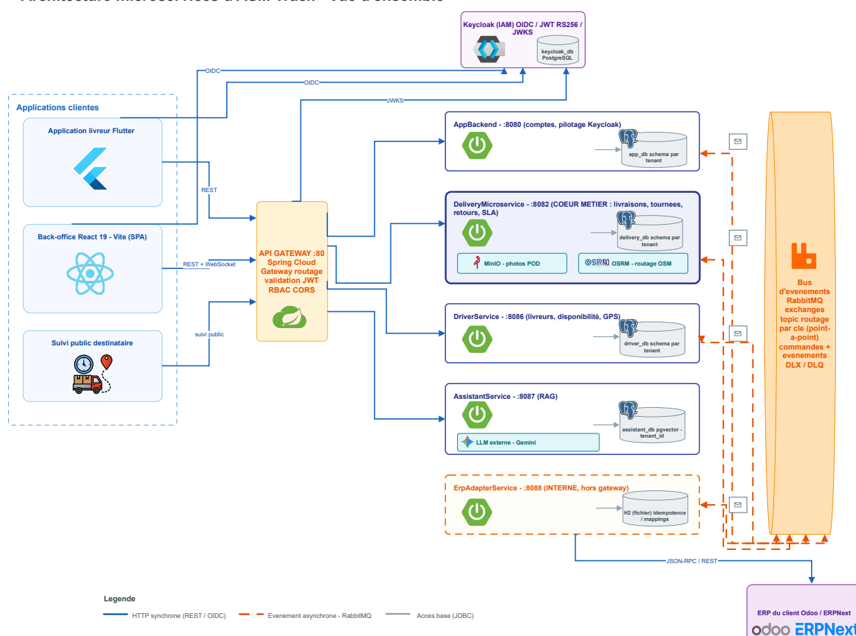
FIG. 3.1 : Vue d'ensemble de l'architecture
