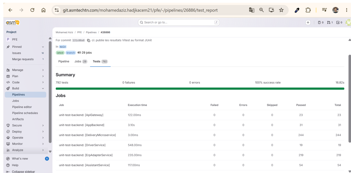
FIG. 9.1 : Rapport de tests agrégé par la chaîne d'intégration
