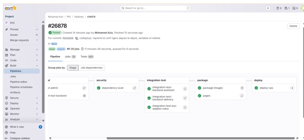
FIG. 9.2 : Les étapes de la chaîne, jusqu'au déploiement
