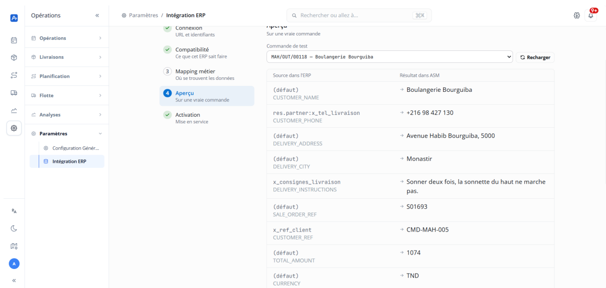
FIG. 5.7 : Aperçu d'une commande avant l'import
