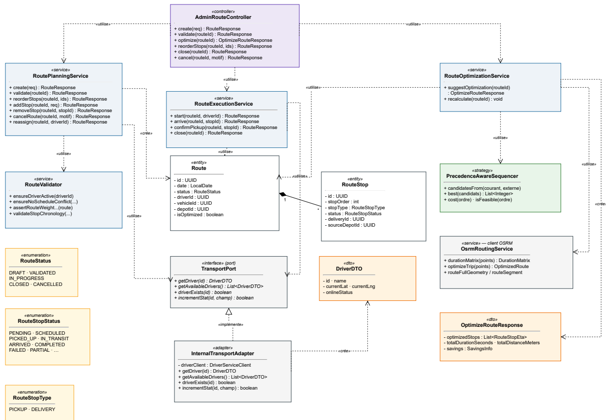
FIG. 6.3 : Classes de conception du sprint 3
