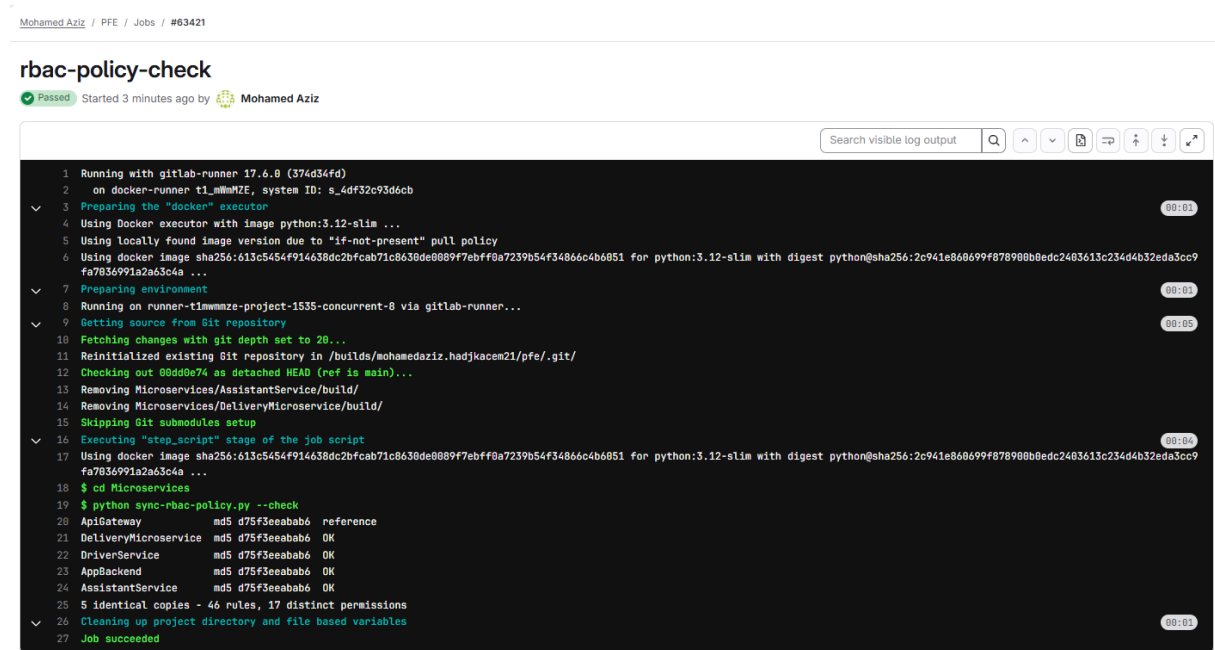
FIG. 4.11 : Contrôle en CI de l'unicité de la politique d'autorisation
