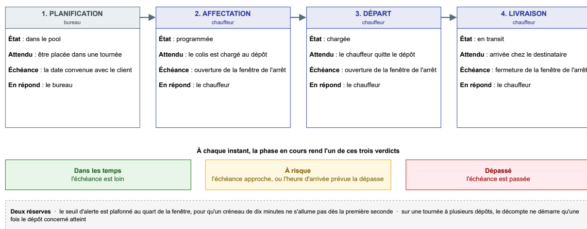
FIG. 6.6 : Les quatre phases d'échéance d'une livraison
