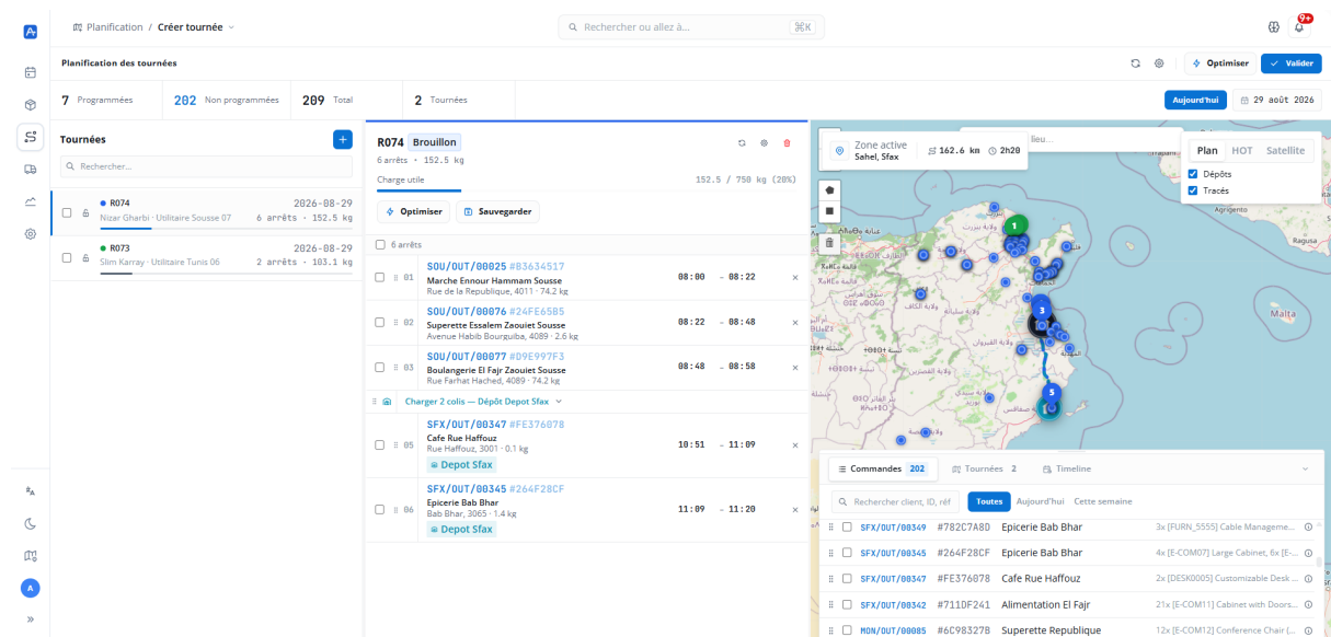
FIG. 6.7 : Planificateur de tournées
