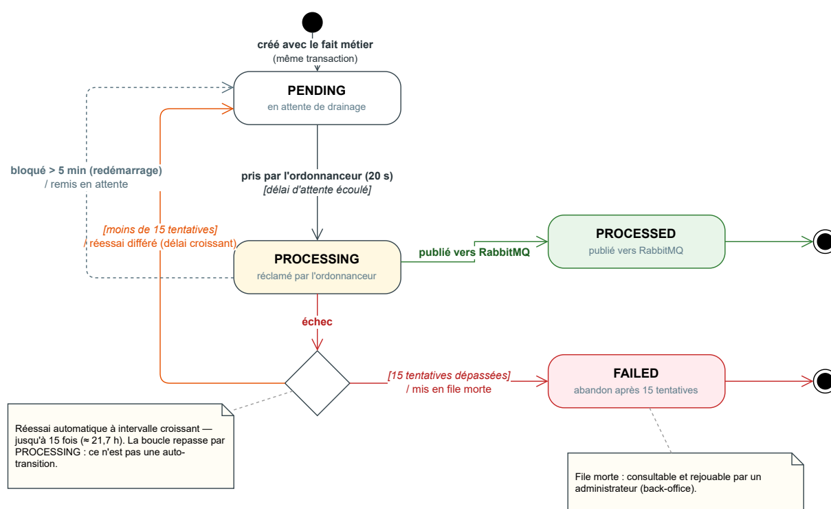
FIG. 5.4 : Automate d'états d'un événement de synchronisation
