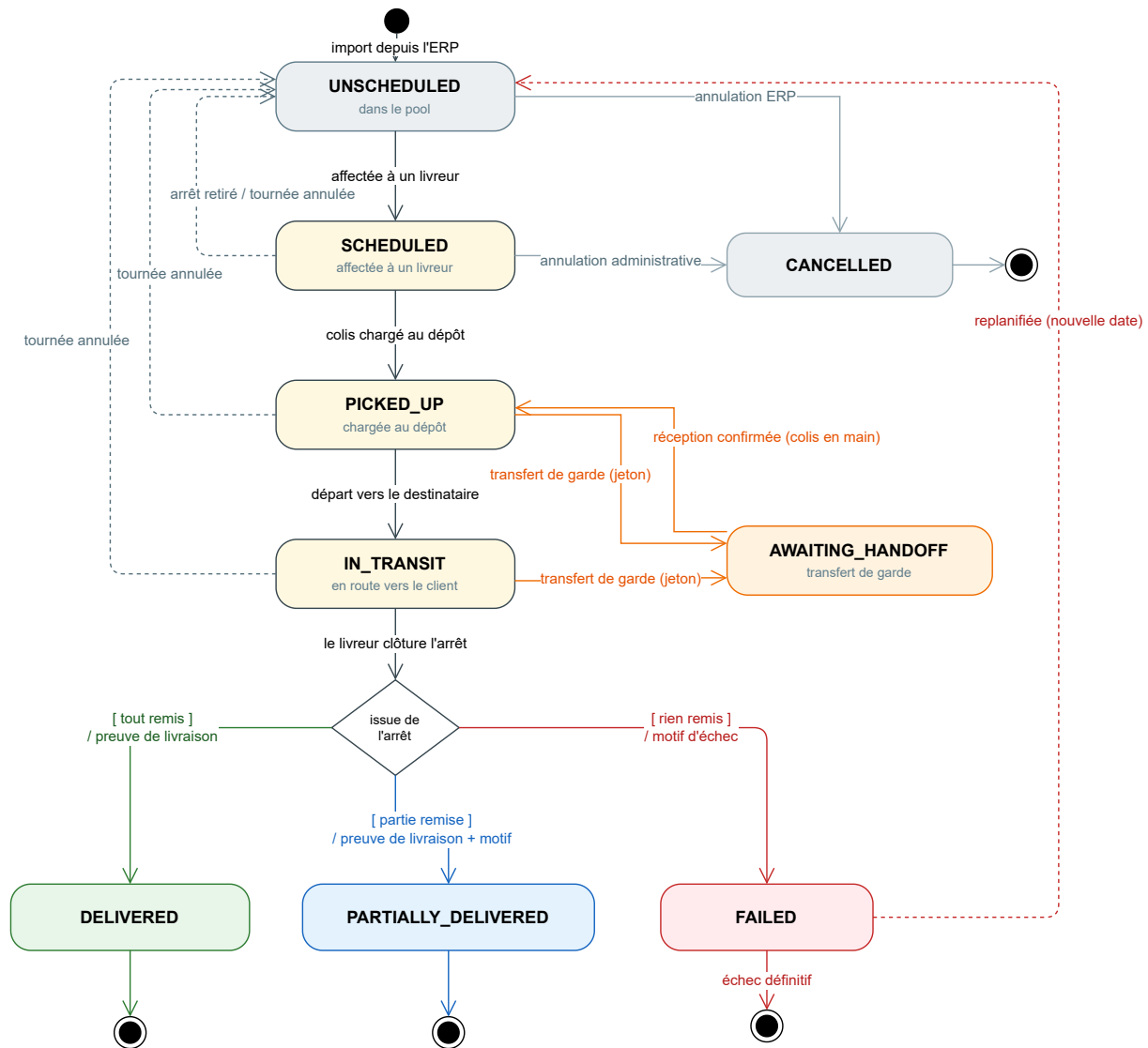
FIG. 6.5 : Machine à états d'une livraison
