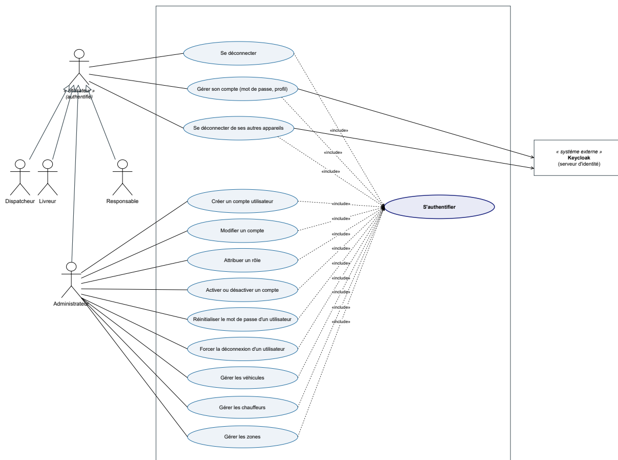
FIG. 4.2 : Diagramme de cas d'utilisation du sprint 1
