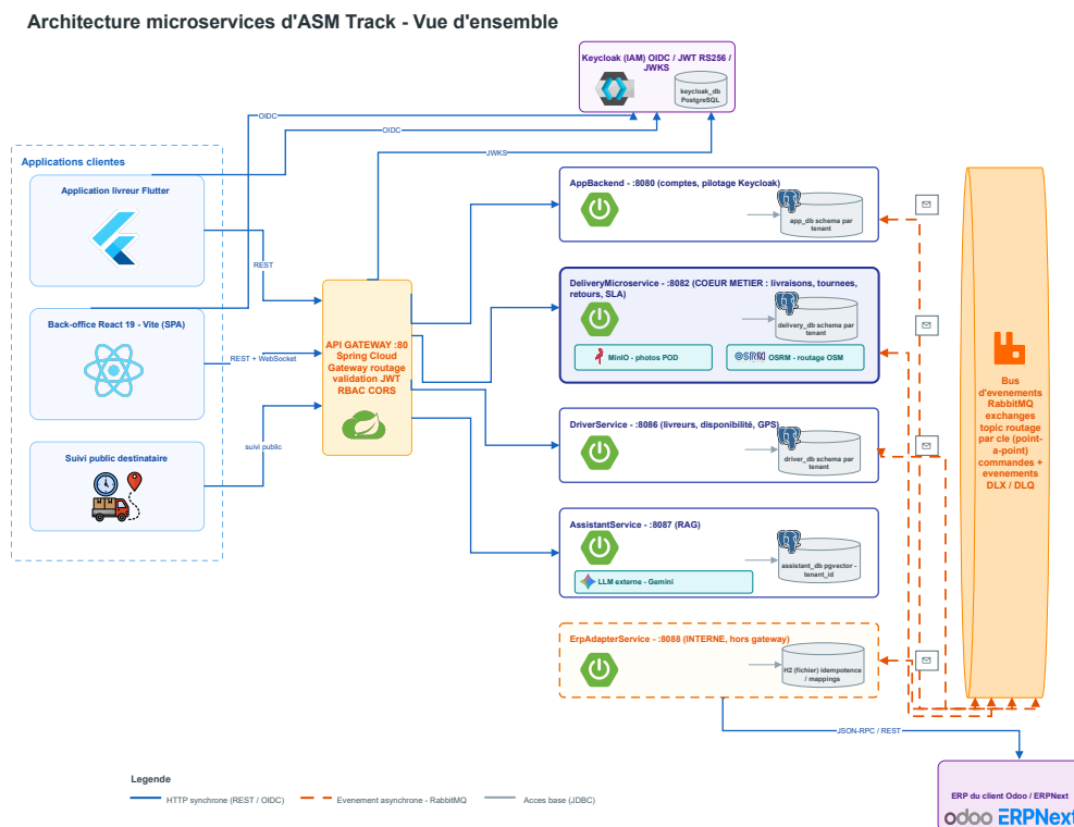
FIG. 3.1 : Vue d'ensemble de l'architecture
