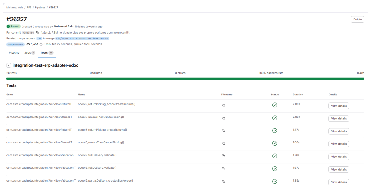
FIG. 5.10 : Exécution en CI de la suite ERP contre deux versions d'Odoo
