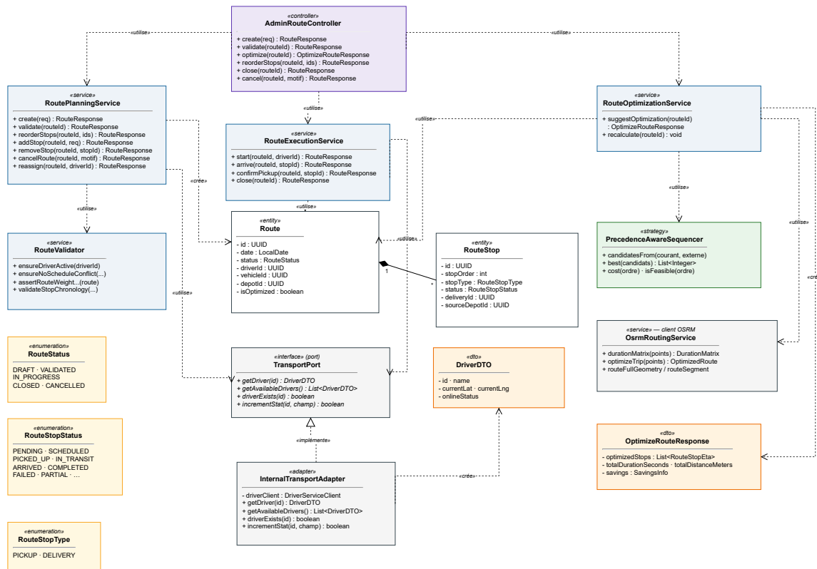
FIG. 6.3 : Classes de conception du sprint 3
