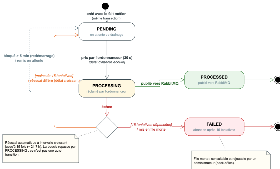
FIG. 5.4 : Automate d'états d'un événement de synchronisation
