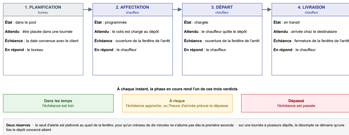
FIG. 6.6 : Les quatre phases d'échéance d'une livraison
