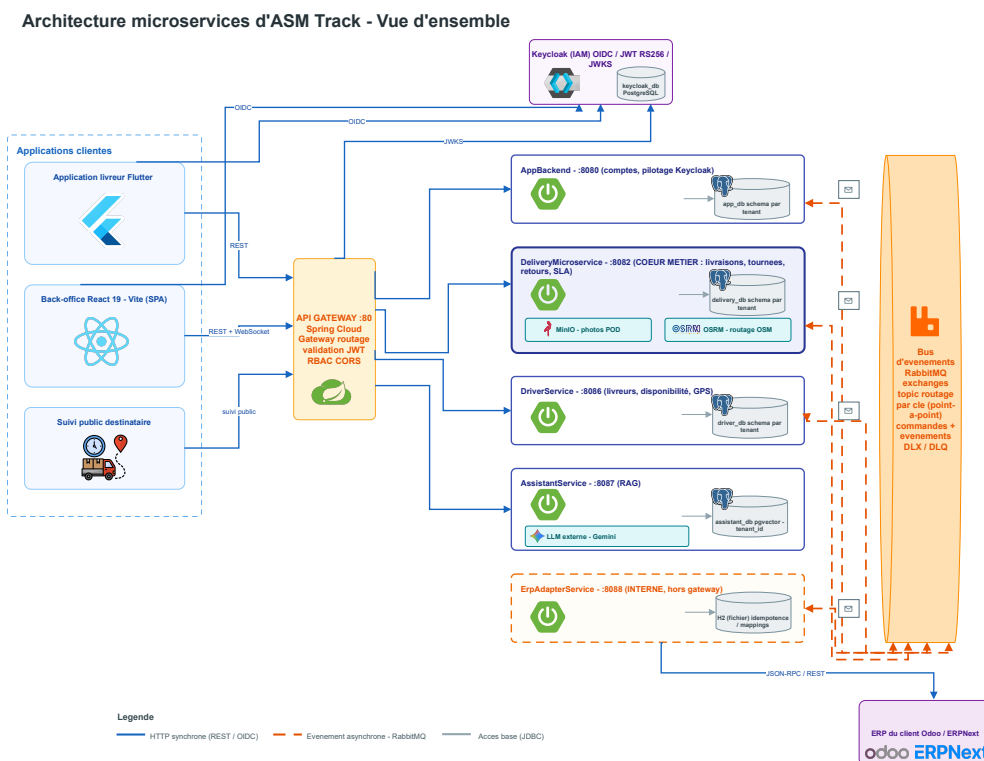
FIG. 3.1 : Vue d'ensemble de l'architecture
