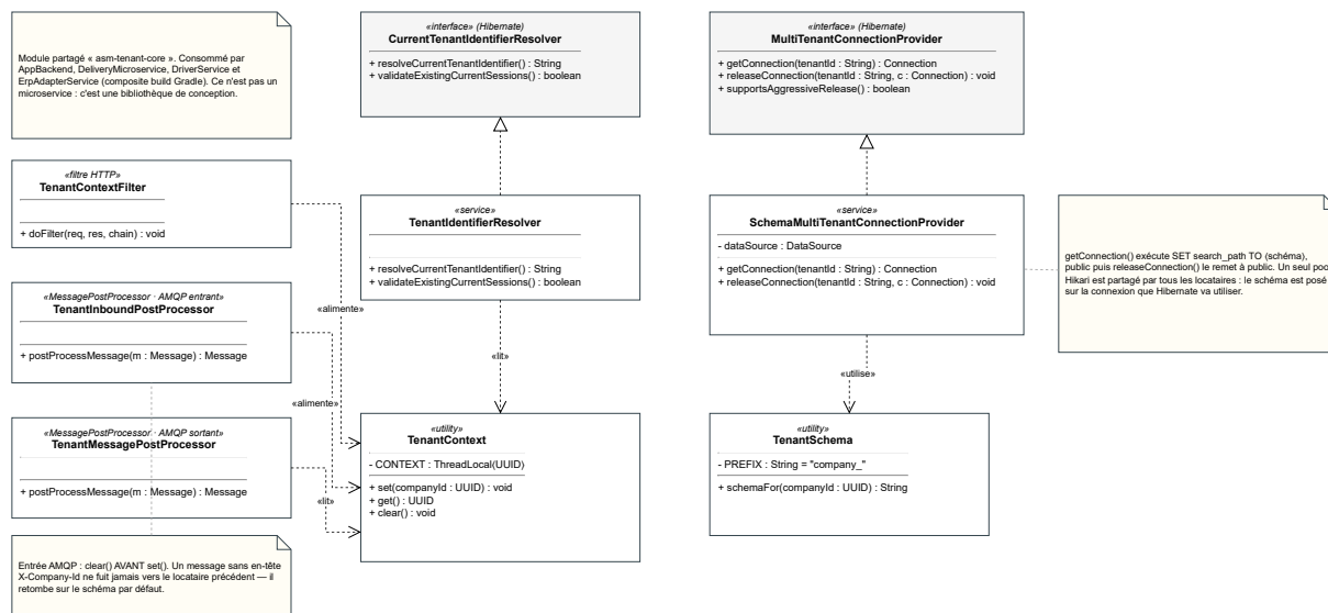
FIG. 4.3 : Diagramme de classes du module asm-tenant-core
