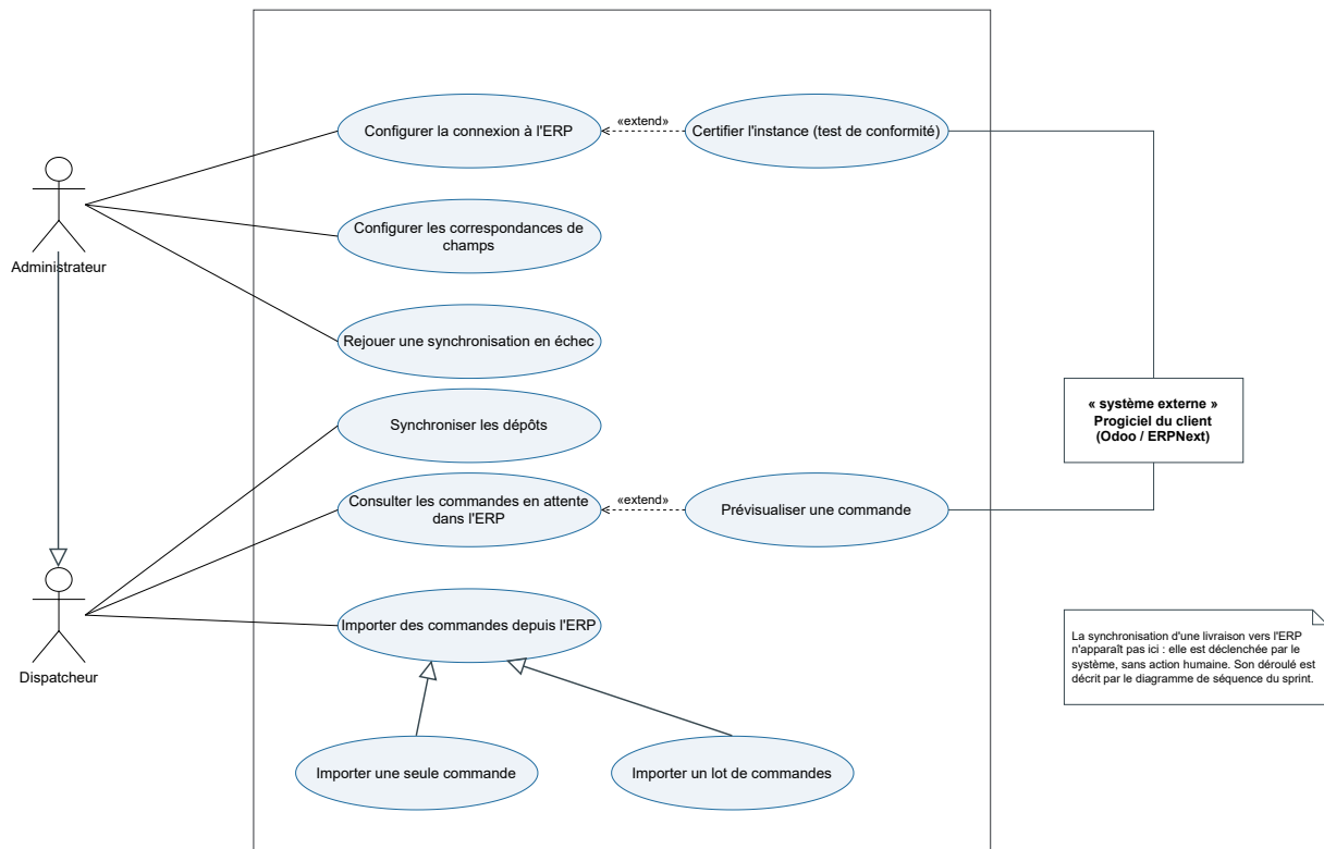
FIG. 5.1 : Diagramme de cas d'utilisation du sprint 2
