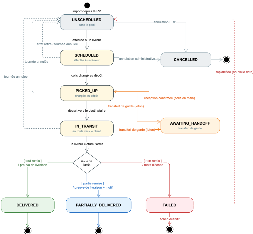
FIG. 6.5 : Machine à états d'une livraison
