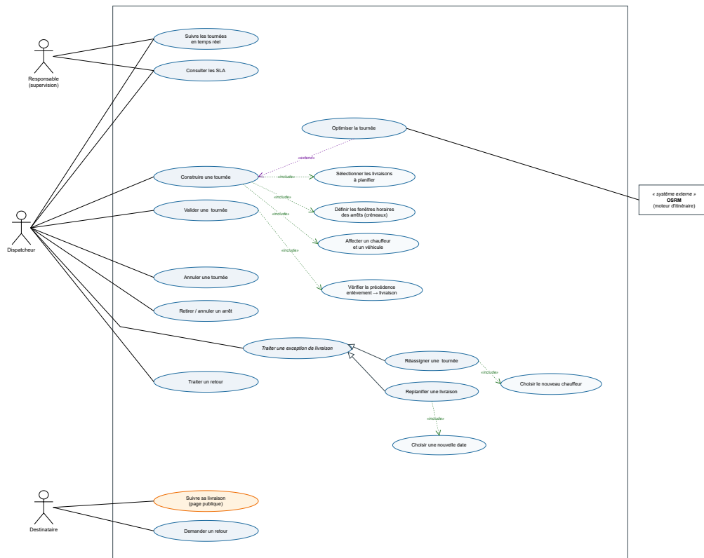
FIG. 6.2 : Diagramme de cas d'utilisation du sprint 3
