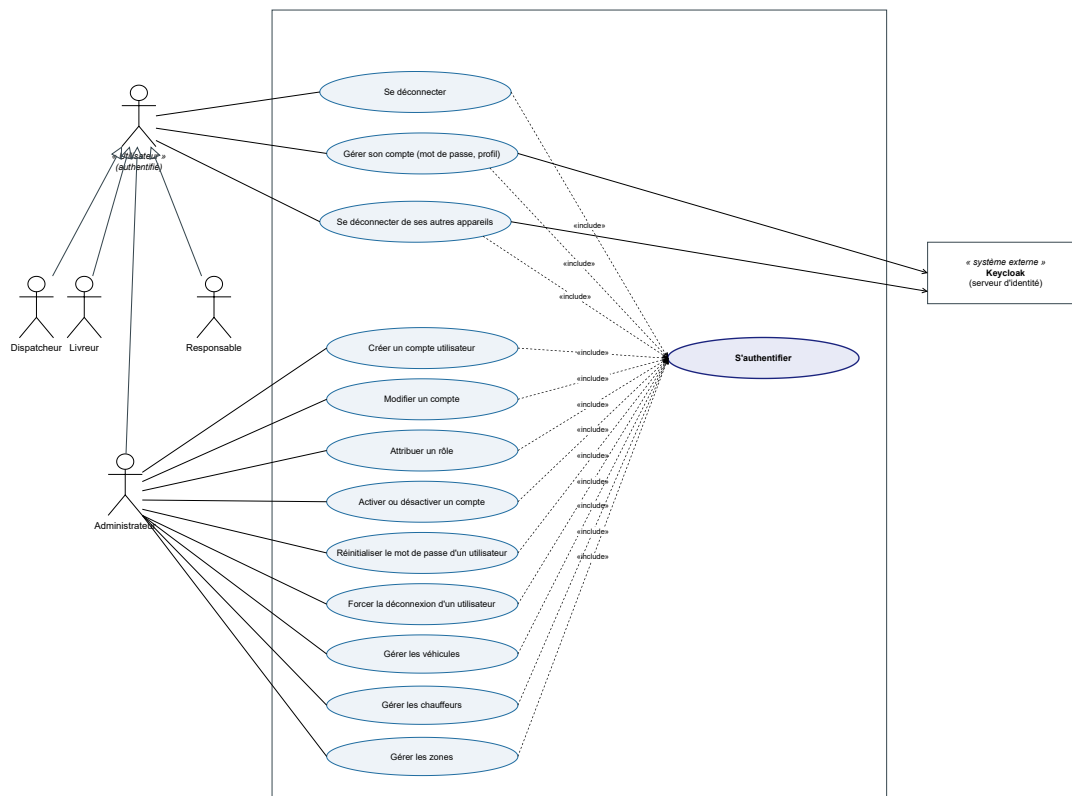
FIG. 4.2 : Diagramme de cas d'utilisation du sprint 1
