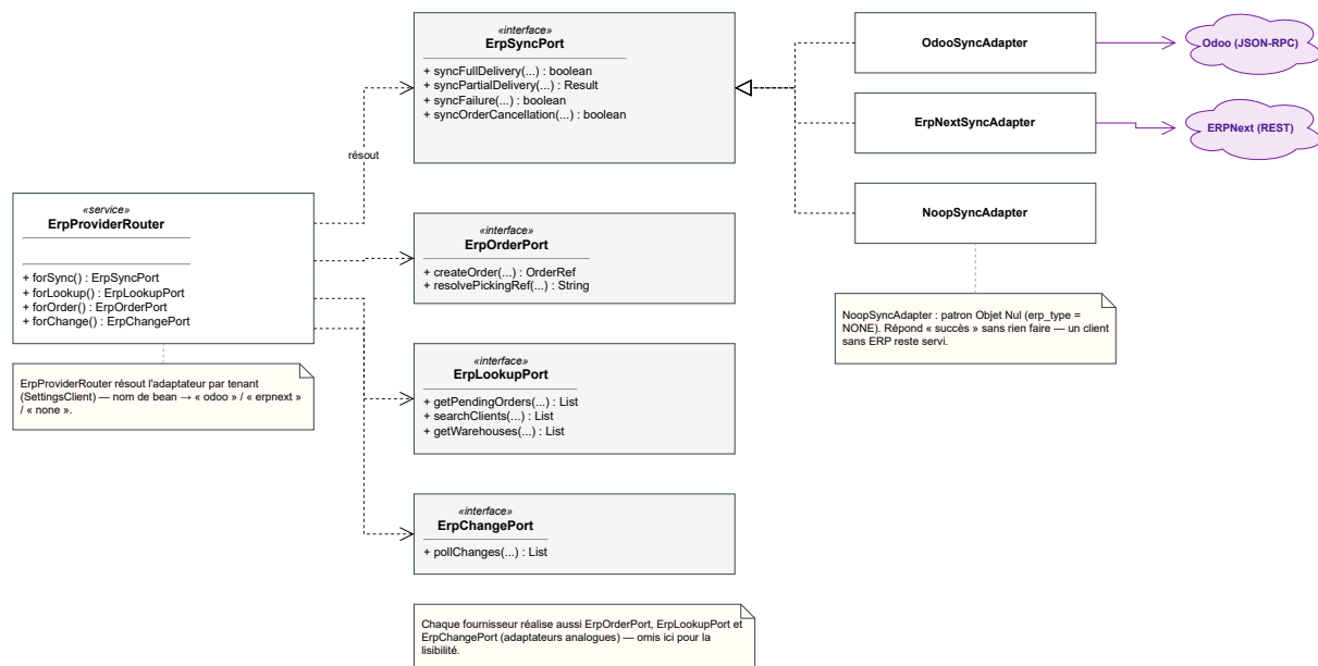
FIG. 5.2 : Ports et adaptateurs de l'intégration ERP
