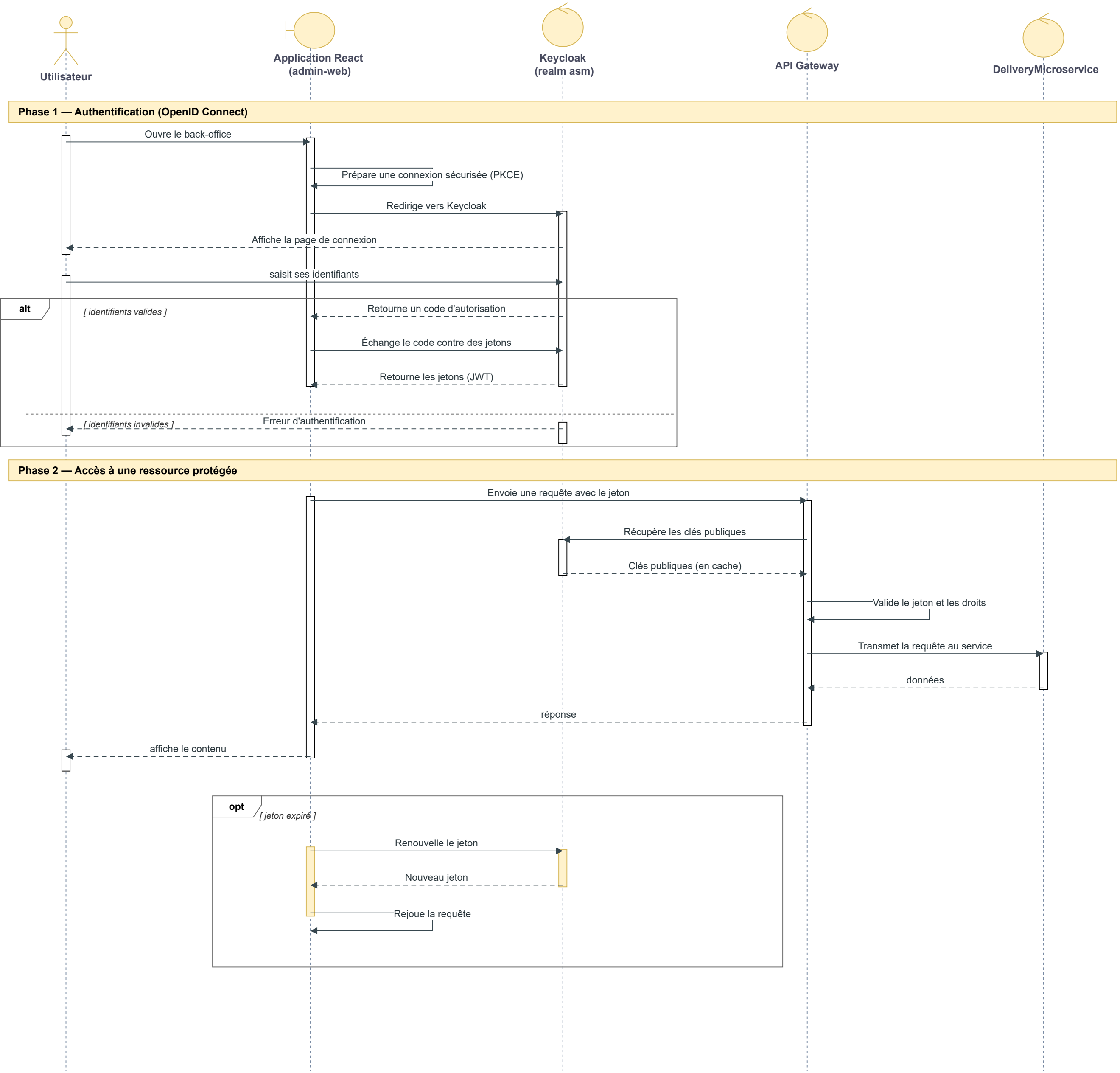
Diagramme de séquence — Authentication OpenID Connect (Keycloak)
