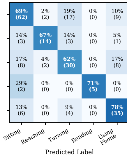
(d) DANN
