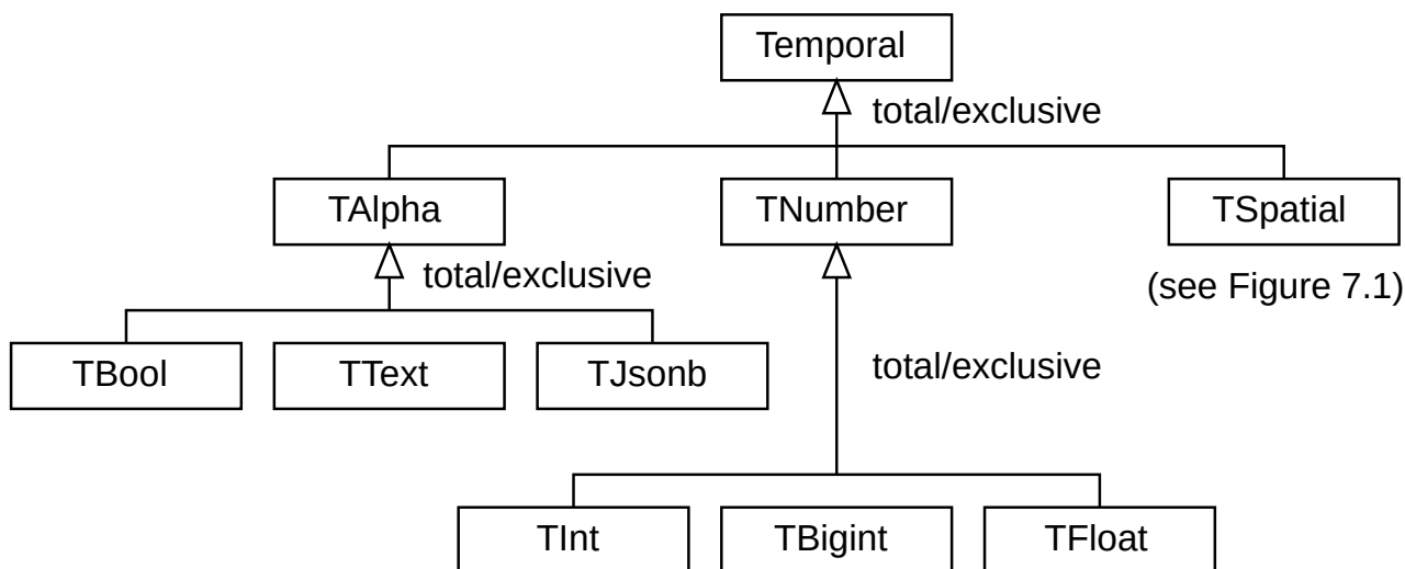
Figura 4.1: Jerarquía de tipos temporales en MobilityDB.
