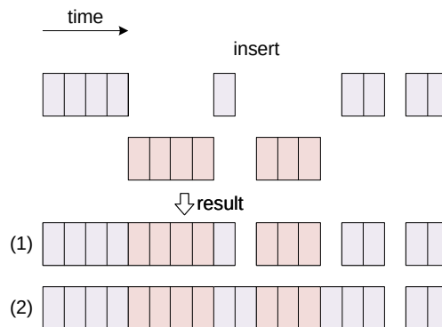
Figura 5.1: Operación de inserción para valores temporales.
