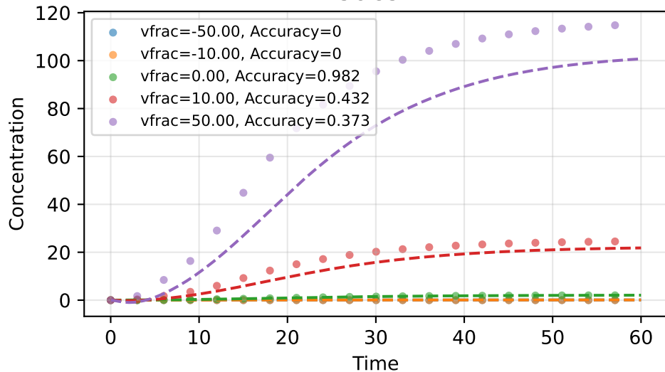
SOCS1
