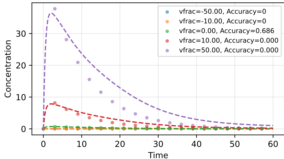
IL7IL7RJAK1
