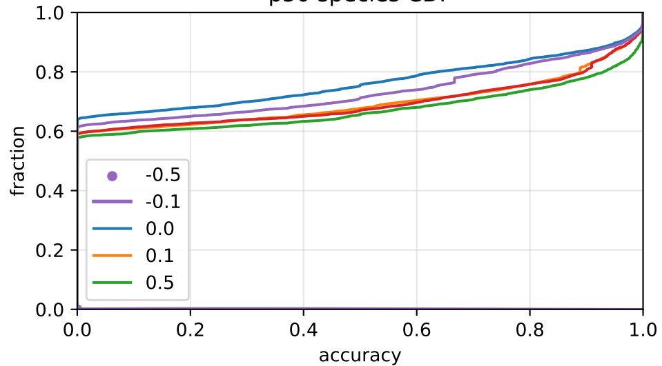
p50 species CDF
