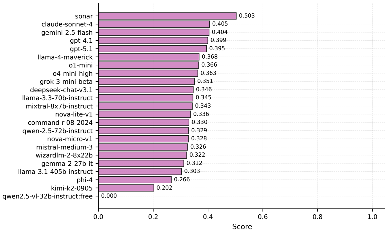
Prompt 2 (P2): MPNet-Mult
