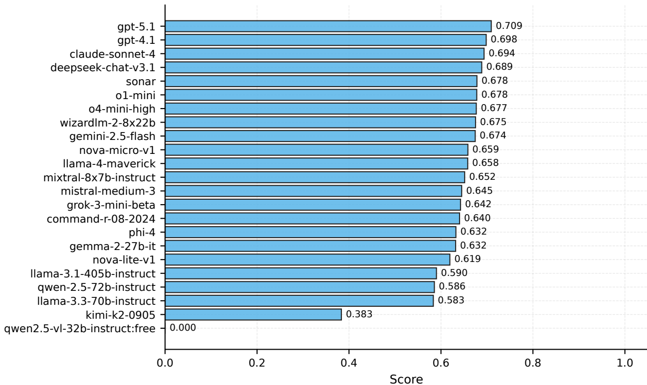
Prompt 2 (P2): SciBETO-mean
