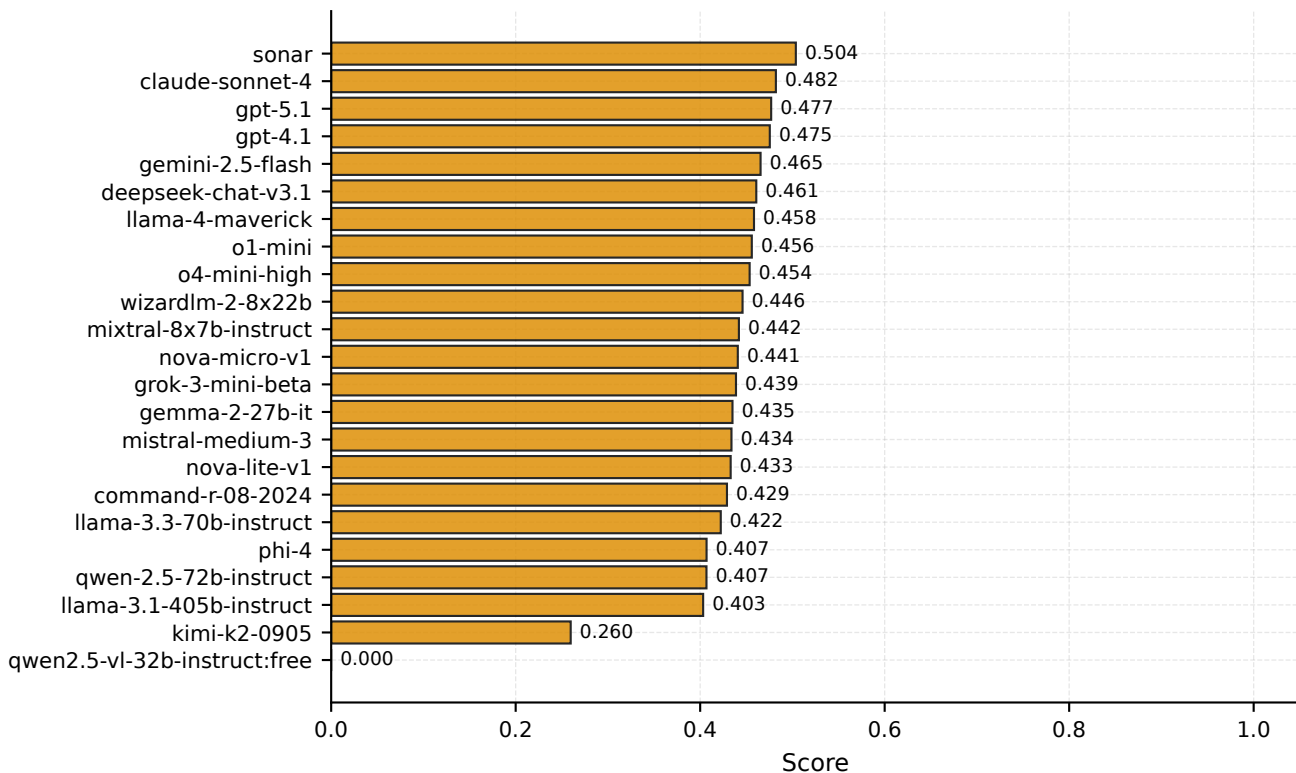
Prompt 2 (P2): BETO F1
