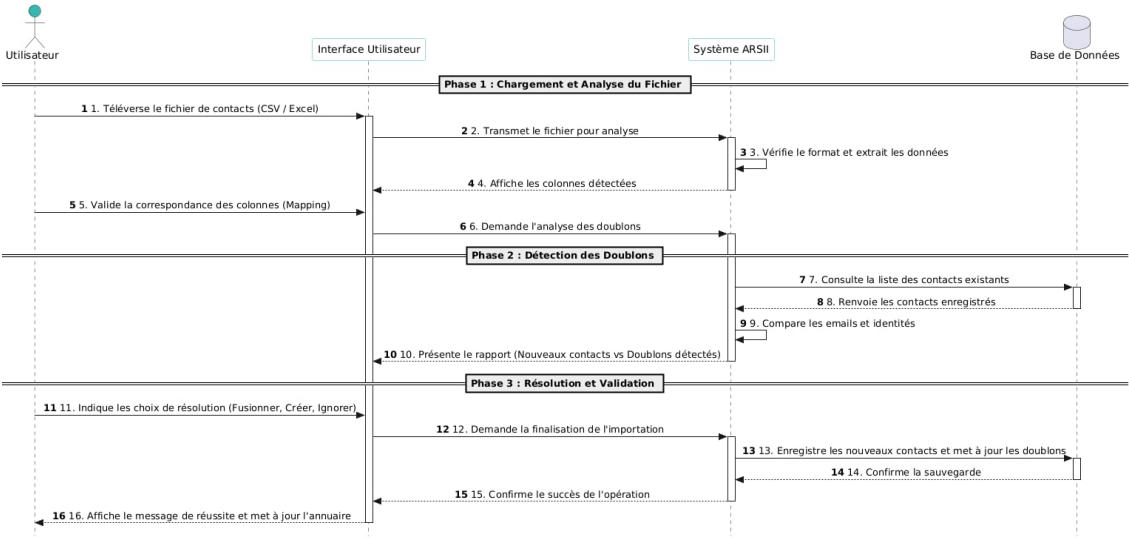
FIGURE 2.3 – Diagramme de séquence — Import de fichier avec gestion des doublons
