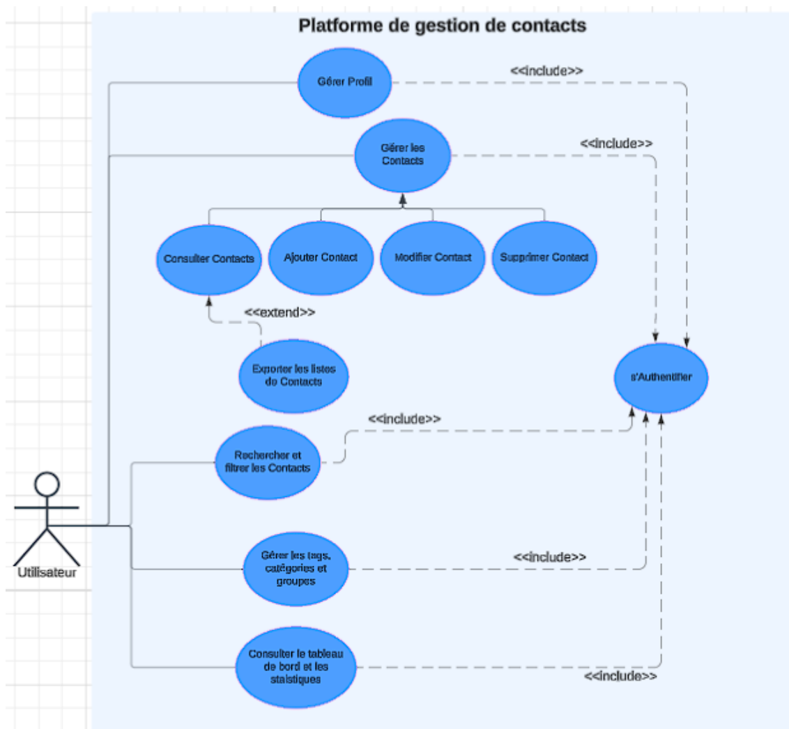
FIGURE 2.1 – Diagramme de cas d'utilisation global
