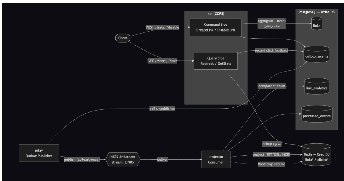
شکل ۱: نمودار مؤلفه‌های سامانه: تفکیک سمت نوشتن (Command) و خواندن (Query)، الگوی Outbox، صف JetStream و Projector.
