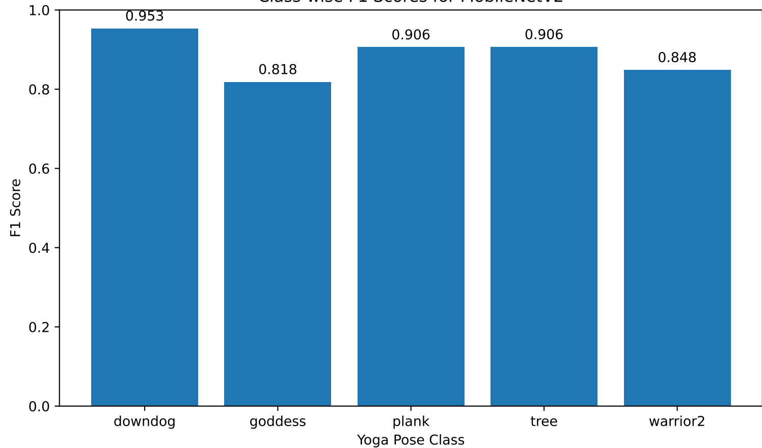
Class-wise F1 Scores for MobileNetV2
